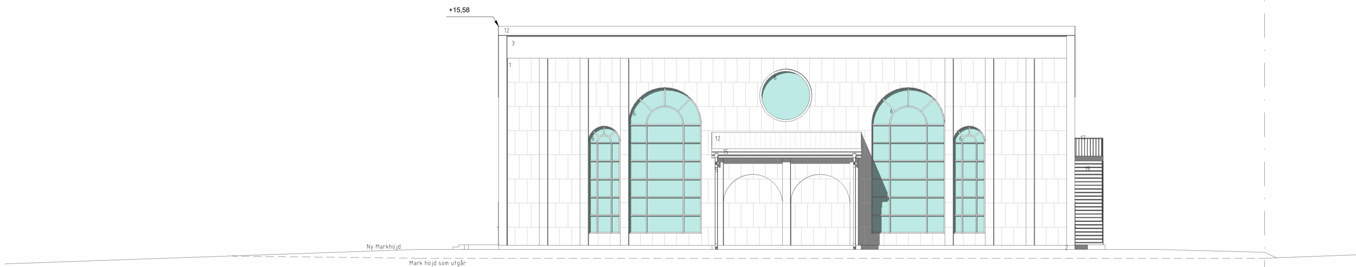
2 Fasad mot sydost 1 : 100
