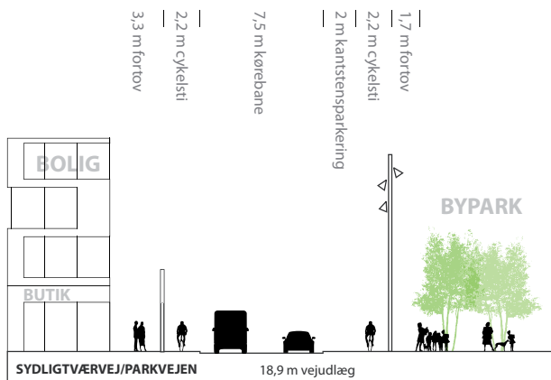
PRINCIP FOR SYDLIGTVÆRVEJ/PARKVEJEN
