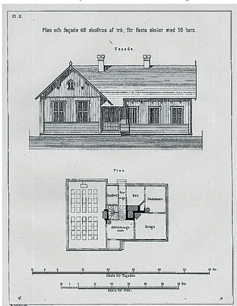
Normalritning – Plan och facade till skolhus af trä, för fasta skolor med 50 barn. Efter riksdagsdebatter under 1850- och 1860-talen om brister i de skolbyggnader som användes runt om i landet, framfördes önskemål om statliga normalritningar. Överintendentämbetet fick uppdraget att ta fram normalritningar och de första publicerades 1865. Läs mer om Västernorrlands skolhus i "Att bygga ett skolväsende, Folkskolans förutsättningar och framväxt 1840–1900" av Johannes Westberg. Finns att ladda ner från Google books.
