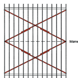
Ved brede, korte bygg kryssavstives hver takflate!
