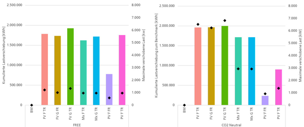
Abbildung 51 Bereitgestellte Flexibilität als verschobene Last zum Benchmark Case in Szenario FREE und CO 2 Neutral
