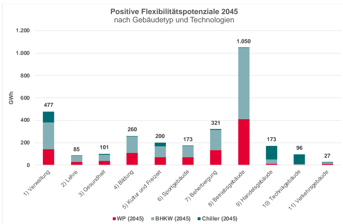
Abbildung 96 Positive Flexibilisierungspotenziale (pFP) in Gigawattstunden (GWh) für das Jahr 2045 (Klimaneutral-Szenario) nach Gebäudekategorie und Technologien
