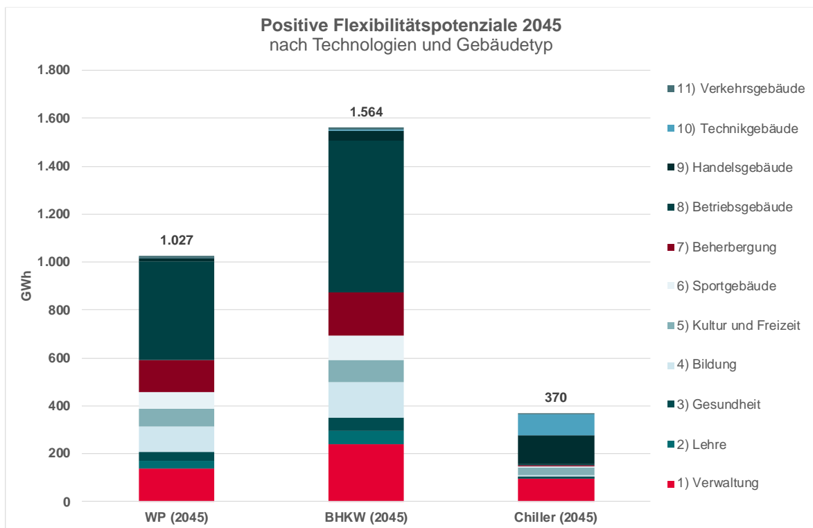
Abbildung 94 Positive Flexibilisierungspotenziale (pFP) in Gigawattstunden (GWh) für das Jahr 2045 (Klimaneutral-Szenario) nach Technologien und Gebäudekategorie
