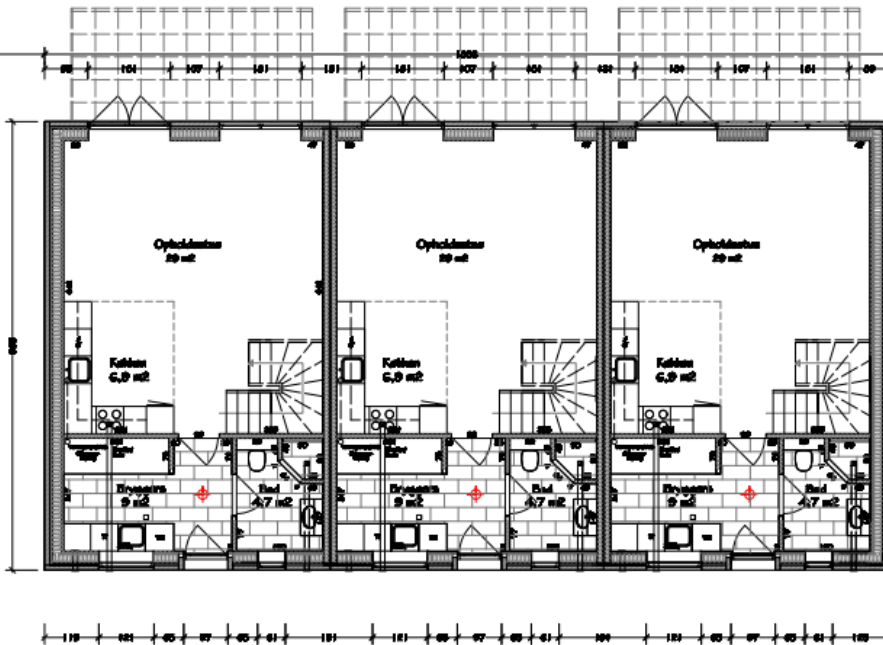
STUEPLAN 1:50
