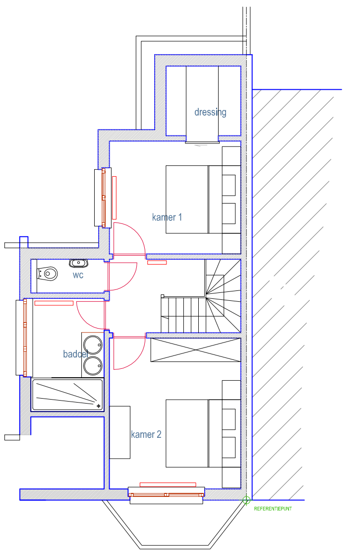
EERSTE VERDIEP
