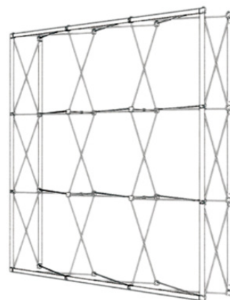
3x3 modul - 224x224x36 cm (BxHxD)
