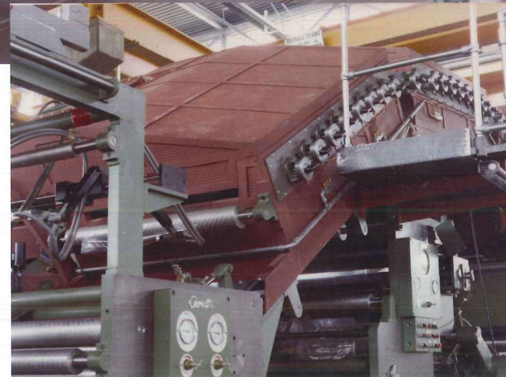
De Cerutti 5 waarop in 7 kleuren kon worden gedrukt. Rechts detailfoto van het droogkanaal dat zorgde voor het versneld drogen na drukken en lamineren
