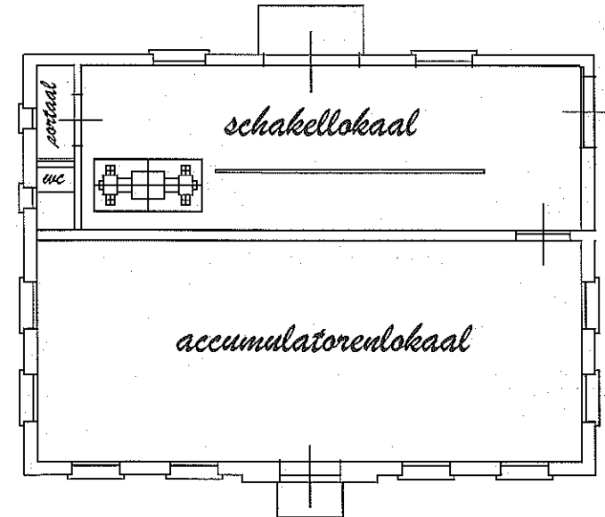
Vooraanzicht en plattegrond accumulatorengedouw
