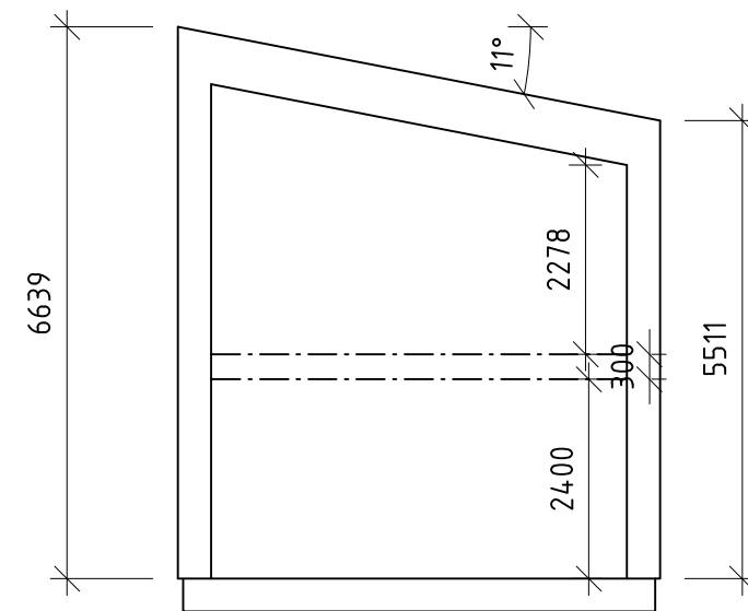
SEKTION A-A
