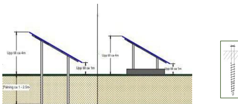
Figur 10, Principskiss av solcellspaneler. Två olika typer av markförankring (fasta system) pålad markförankring samt fristående markförankring. Exempel på "jordborr" till höger.
