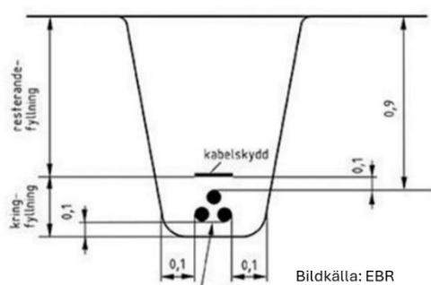
Figur 11. Principskiss kabelgrav
