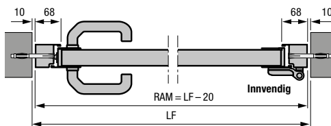
Sidedør med blokkarm av aluminium, profiltipe 2 Montering i åpningen
