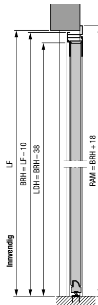
Sidedør med hjørnekarm av aluminium profiltipe 2 Utvendig montering
