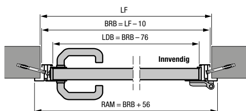
Sidedør med hjørnekarm av aluminium profiltipe 1 eller 2 Innvendig montering
