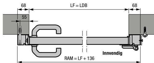
Sidedør med blokkarm av aluminium, profiltipe 1 Montering bak åpningen
