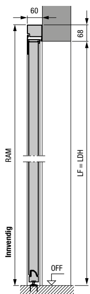
Sidedør med blokkarm av aluminium, profiltipe 2 Montering bak åpningen
