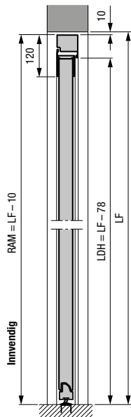
Sidedør med blokkarm av aluminium, profiltipe 2 Montering i åpningen
