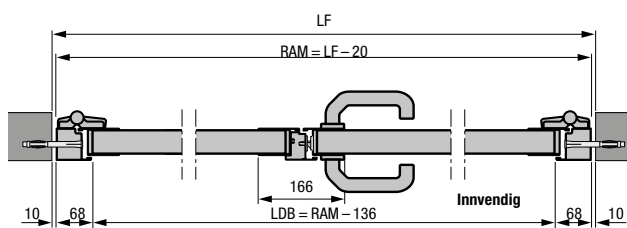
2-fløyet sidedør med blokkarm av aluminium, profiltipe 2 Montering i åpningen
