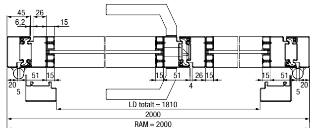
Horizontalt tverrsnitt 2-fløyet interiørdør
