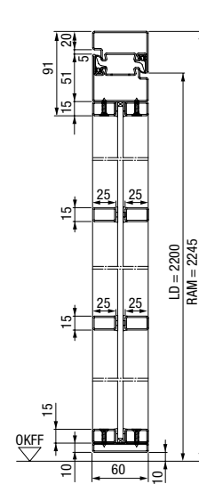
Vertikalt tverrsnitt 1-fløyet interiørdør
