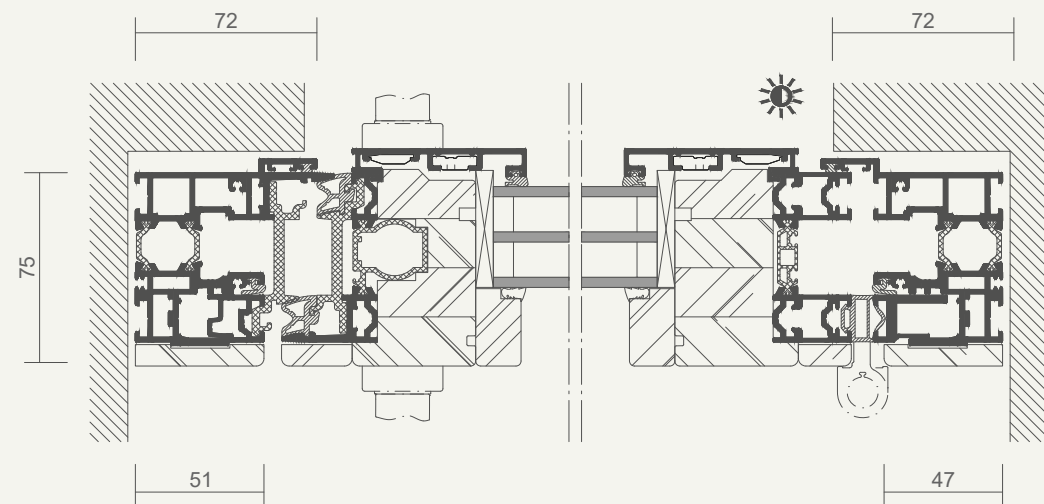
Horizontalsnitt
