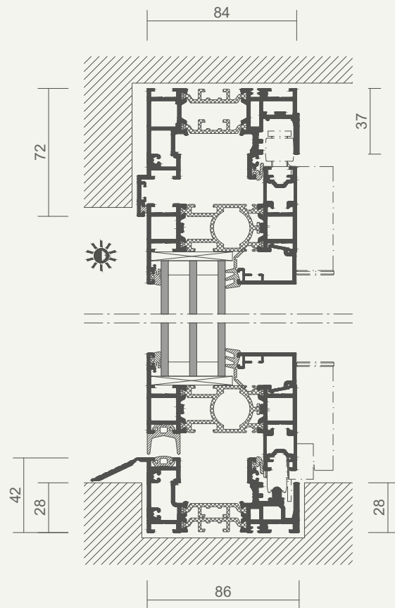
Vertikalsnitt
