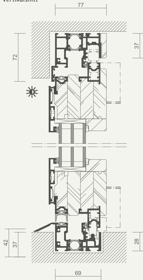
Vertikalsnitt
