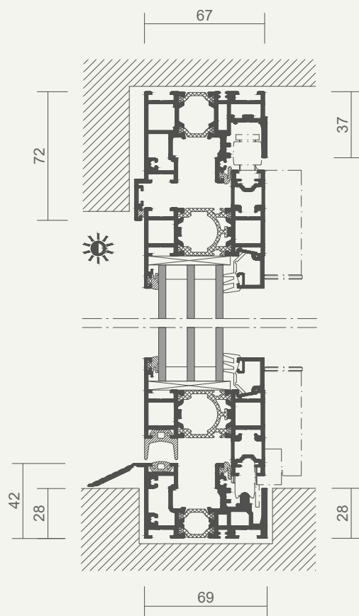
Vertikalsnitt
