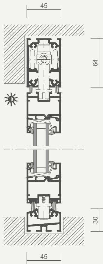
Vertikalsnitt
