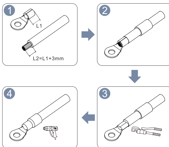
Figura 21 - Crimpatura terminali OT
