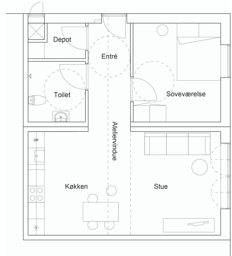
Plantegning af Boligtype D2_A
