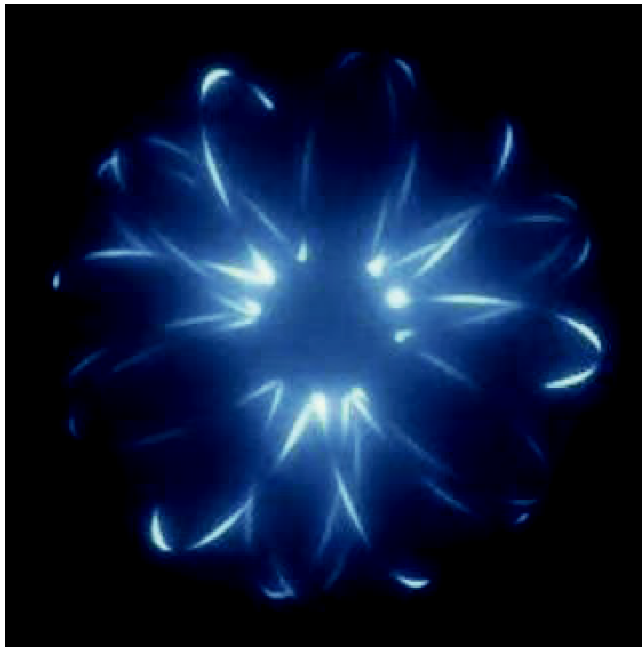
Photons
