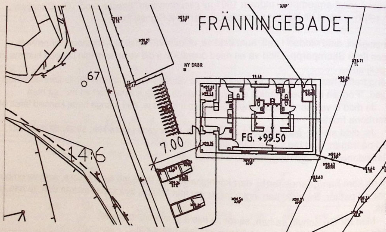
Ritning över nya entrén med cykelställ, handikapparkering, kiosk och omklädningsrum.
