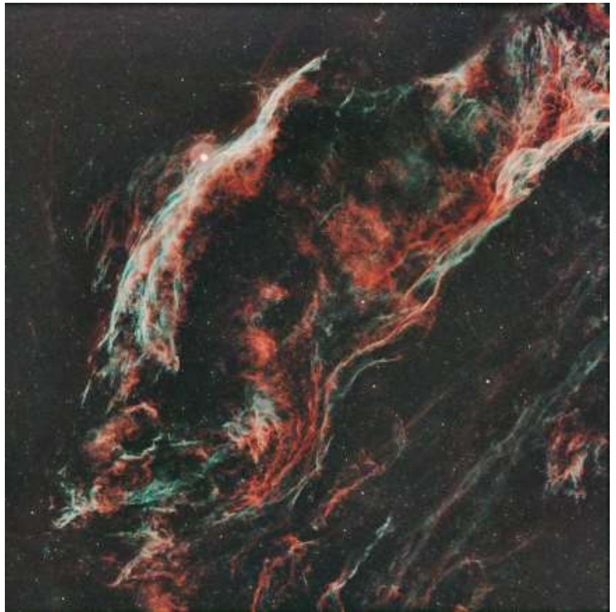
Een nova restant. Dit blijft over nadat een ster explodeert. NGC 6992 laat enorm veel waterstof, zwavel en zuurstof na. Daar kan weer een nieuwe ster uit voortkomen.
