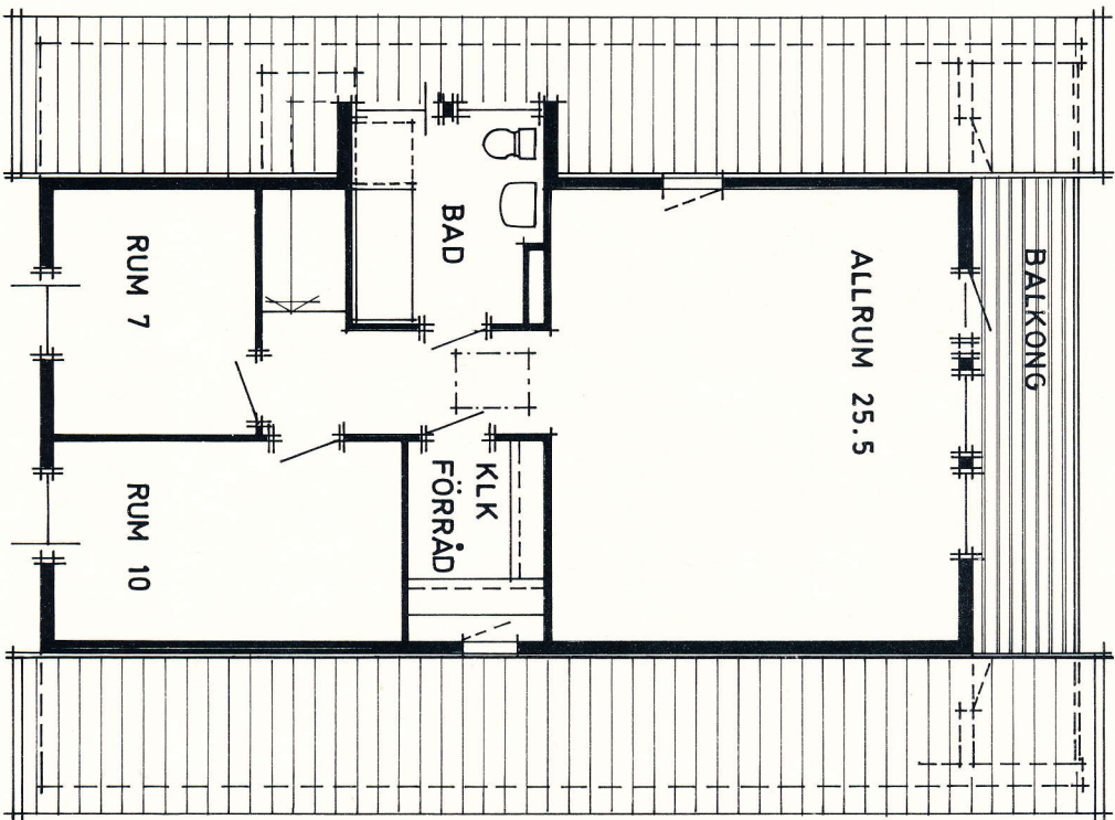
ÖVERPLAN
