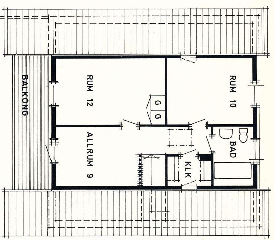
ÖVERPLAN
