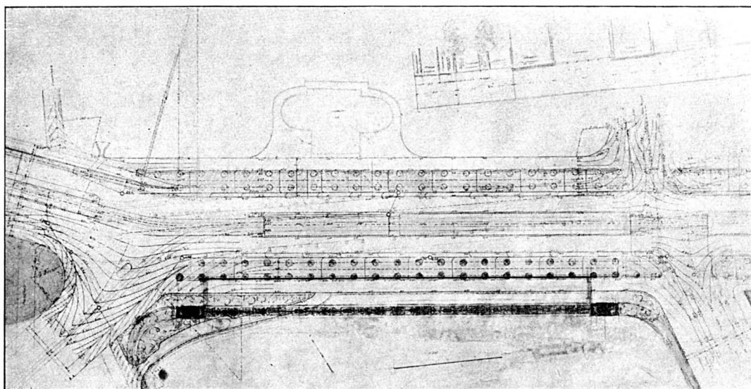
Situationsplan. Tilvenstre Aaboulevardens og Rosenørns Allés Indføring i Gyldenløvesgade. Foroven Pebblingesø; forneden Sct. Jørgens Sø.
