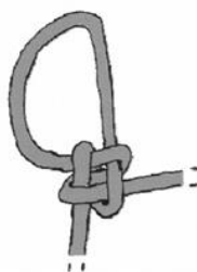
Vänskapsknopen
