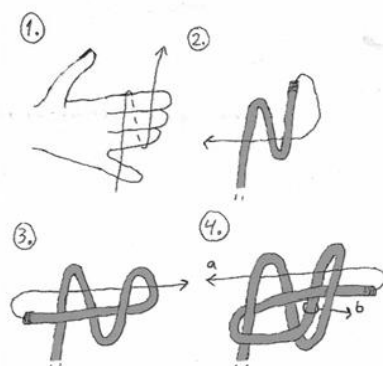
Vänskapsknopen
