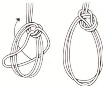
Dubbel pålstek
