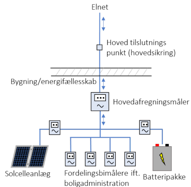
Figur 2 - Principskitse af elnettet i et energifællesskab
