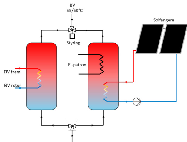
Figur 55 - Principskitse af et solvarmeanlæg i samspil med fjernvarme. Solfangerne opvarmer vand i en beholder udstyret med en el-patron.
