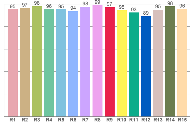
CRI: 96,5 (R1-R8)
