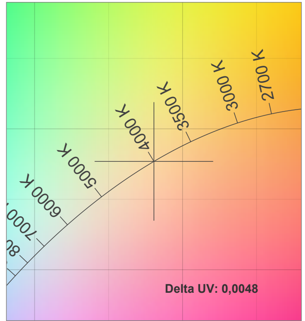
CRI: 96,5 (R1-R8)
