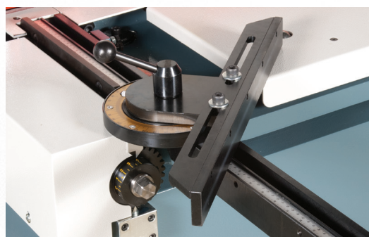
Verstellbarer Winkelanschlag 0-180°
