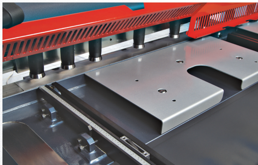
Hochklappbarer Fingerschutz Kugeltisch Hydraulische Niederhalter
