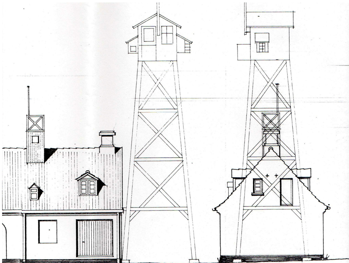
FACADE ØST.
