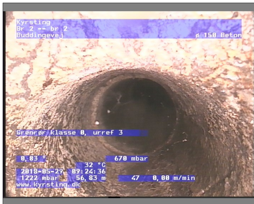
Foto: Br 2-br 209244633-29-05-18_A.JPG, Medie #:: De Engelske _0, 00:01:41 56,83m, Grenør klasse 0, urref 3
