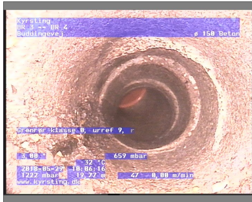
Foto: BR 3-BR 410062614-29-05-18_A.JPG, Medie #:: De Engelske _0, 00:05:50 19,77m, Grenrør klasse 0, urref 9 / rb 2 i gren
