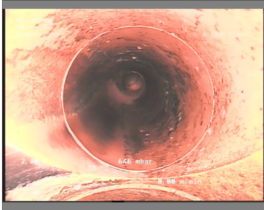
Foto: 16-171059343-29-05-18_A.JPG, Medie #.: De Engelske _0, 00:01:20 1,35m, Grenrør klasse 0, urref 10
