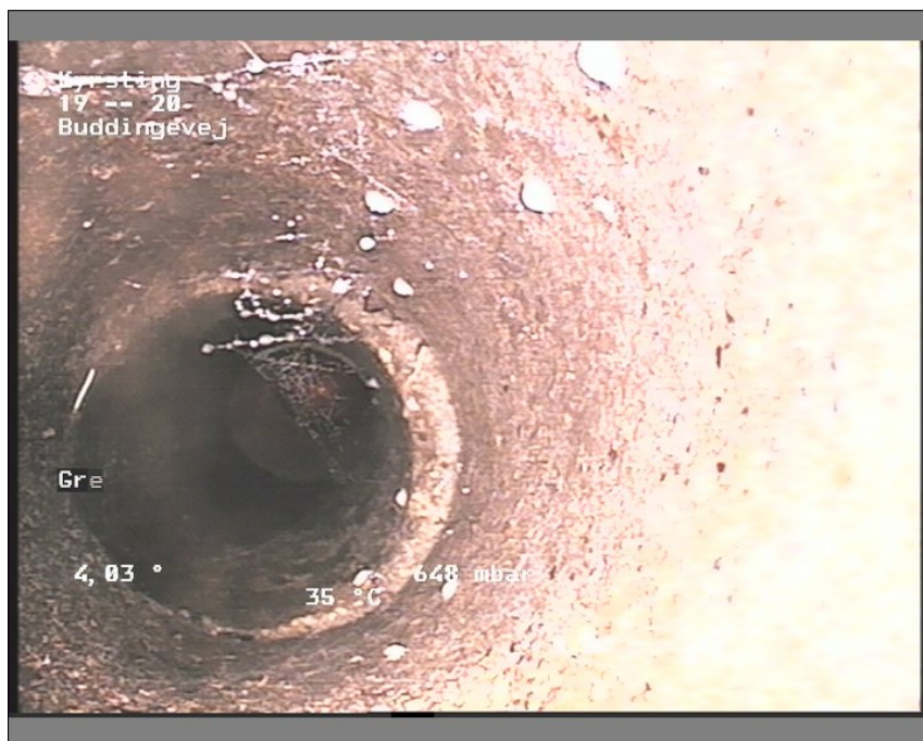
Foto: 19-2012512213-29-05-18_A.JPG, Medie #:: De Engelske _0, 00:02:38 43,88m, Grenrør klasse 0, urref 9
