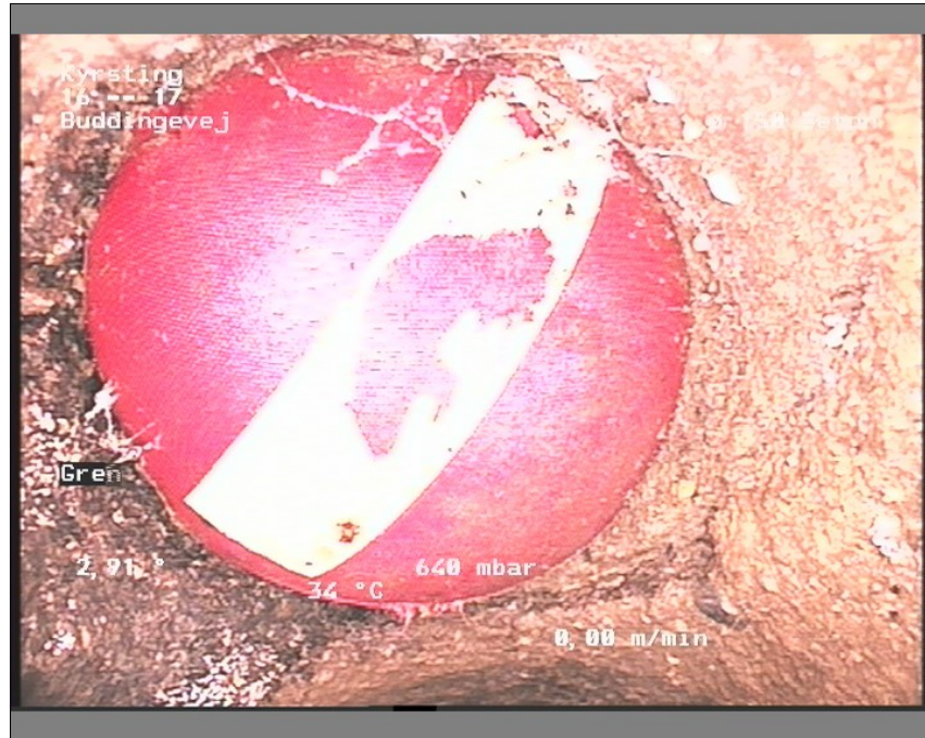
Foto: 16-1711265122-29-05-18_A.JPG, Medie #:: De Engelske _0, 00:00:37 15,46m, Grenrør klasse 0, urref 10, Stiktilslutning er afproppet / Rotte stop prop
