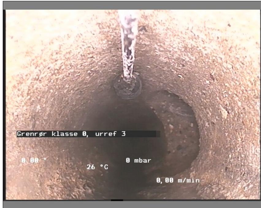
Foto: br 10-br 111335209-29-05-18_A.JPG, Medie #.: De Engelske _0, 00:03:55 26,33m, Grenrør klasse 0, urref 3
