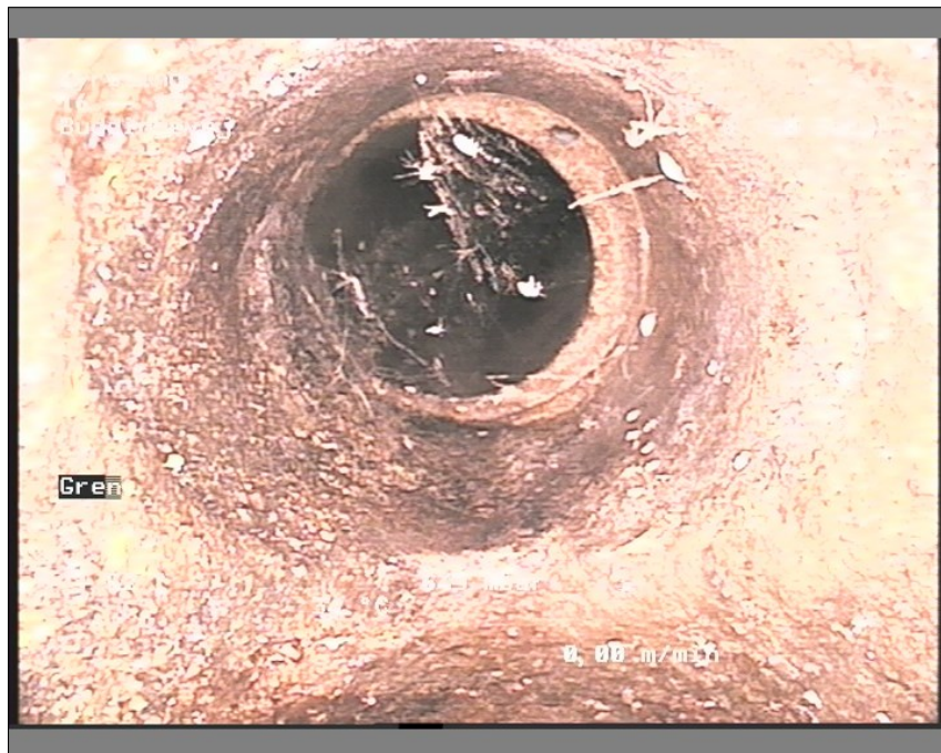
Foto: 16-1711291728-29-05-18_A.JPG, Medie #:: De Engelske _0, 00:00:37 22m, Grenrør klasse 0, urref 10 / fs 3 i tilslutning
