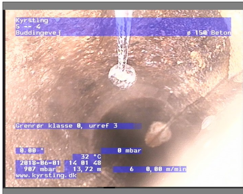
Foto: 4-514020412-29-05-18_A.JPG, Medie #:: De Engelske _0, 00:03:06 13,72m, Grenrør klasse 0, urref 3
