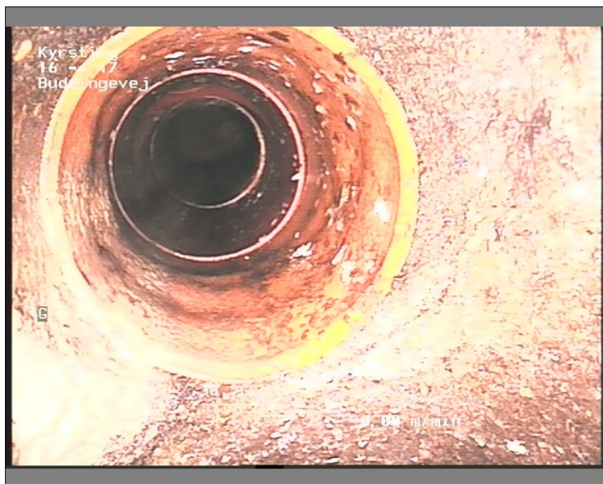
Foto: 16-1711260821-29-05-18_A.JPG, Medie #:: De Engelske _0, 00:00:37 15,07m, Grenrør klasse 0, urref 10
