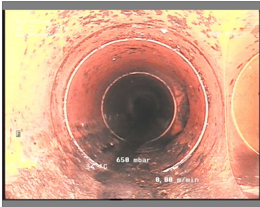
Foto: br 21-21a1350049-29-05-18_A.JPG, Medie #:: De Engelske _0, 00:01:01 13,49m, FS3, Forskudt samling
