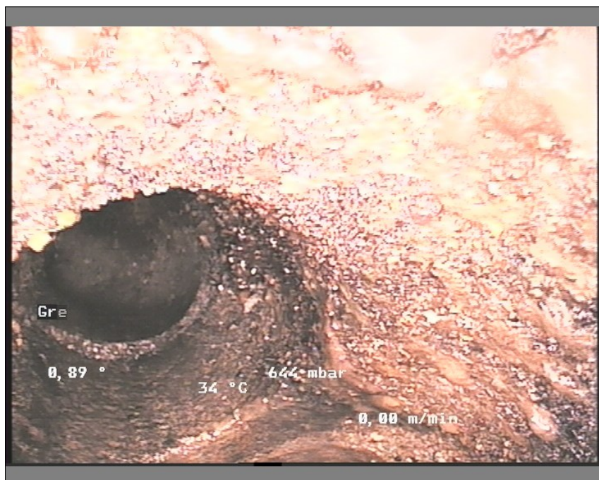
Foto: br 17-br 1812100042-29-05-18_A.JPG, Medie #.: De Engelske _0, 00:14:22 31m, Grenrør klasse 0, urref 11
