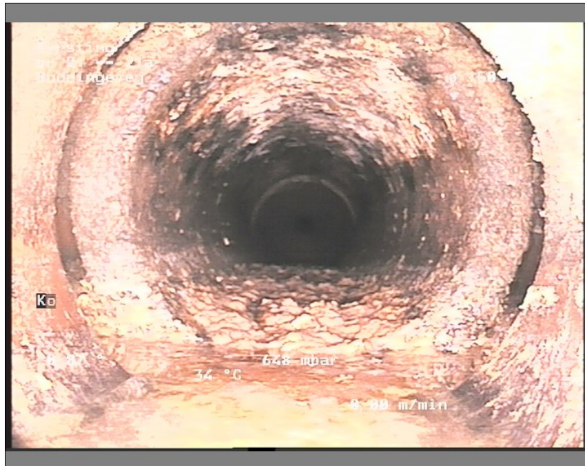
Foto: br 21-21a14010925-29-05-18_A.JPG, Medie #.: De Engelske _0, 00:06:13 27,41m, Konstruktionsændring klasse 4, Materialeændring, Dimensionsændring
