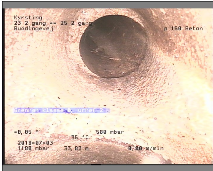
Foto: 23 2 gang-25 2 gang09340519-29-05-18_A.JPG, Medie #: De Engelske _0, 00:09:01 33,83m, Grenrør klasse 0, urref 2
