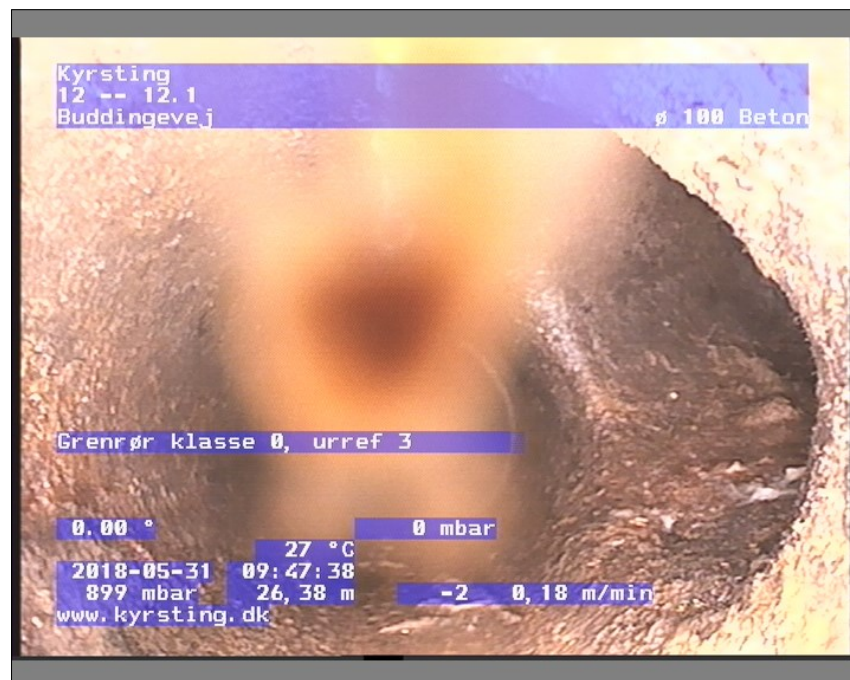
Foto: 12-12.109475424-29-05-18_A.JPG, Medie #: De Engelske _0, 00:12:47 26,39m, Grenrør klasse 0, urref 3
