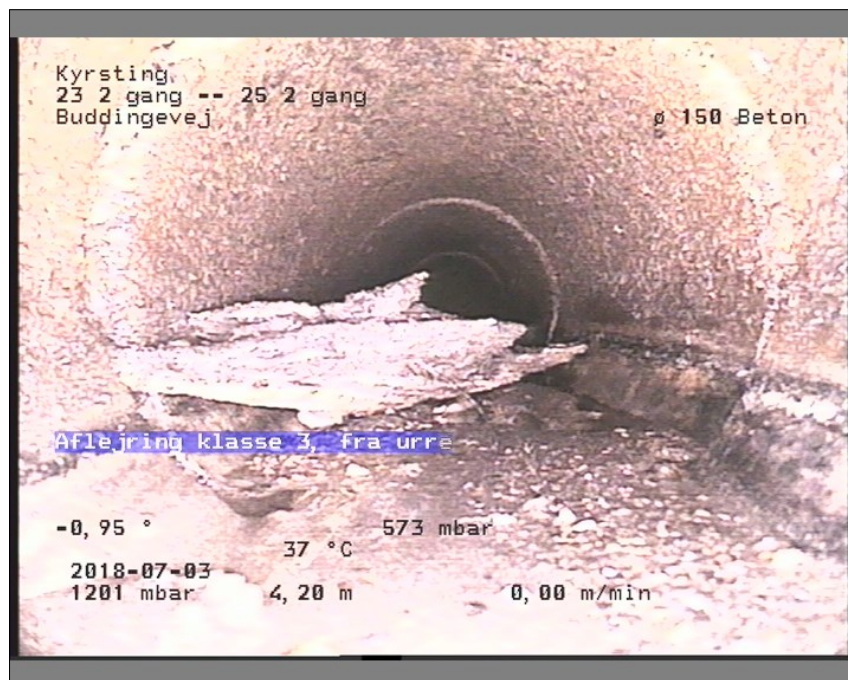
Foto: 23 2 gang-25 2 gang0900026-29-05-18_A.JPG, Medie #: De Engelske _0, 00:01:29 4,2m, Aflejring klasse 3, fra urref 5 til urref 8, Hårde materialer
