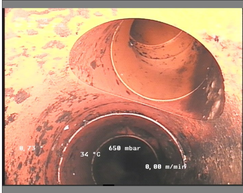
Foto: br 21-21a1349468-29-05-18_A.JPG, Medie #:: De Engelske _0, 00:01:01 13,49m, Grenrør klasse 0, urref 3
