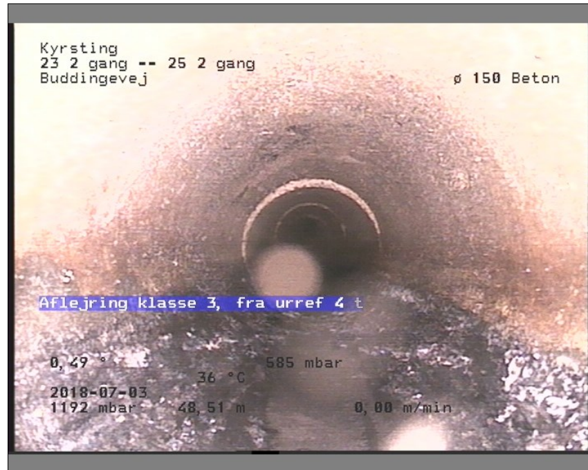
Foto: 23 2 gang-25 2 gang09385227-29-05-18_A.JPG, Medie #: De Engelske _0, 00:12:02 48,51m, Aflejring klasse 3, fra urref 4 til urref 8, Hårde materialer, Start
