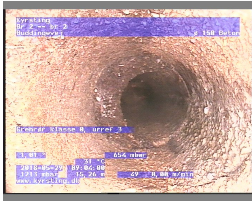
Foto: Br 2-br 209041012-29-05-18_A.JPG, Medie #:: De Engelske _0, 00:01:41 15,26m, Grenrør klasse 0, urref 3
