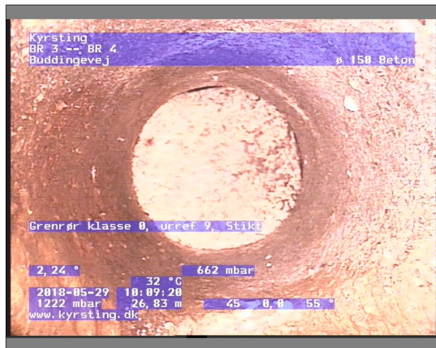
Foto: BR 3-BR 410093019-29-05-18_A.JPG, Medie #: De Engelske _0, 00:07:55 26,83m, Grenrør klasse 0, urref 9, Stiktilslutning er afproppet
