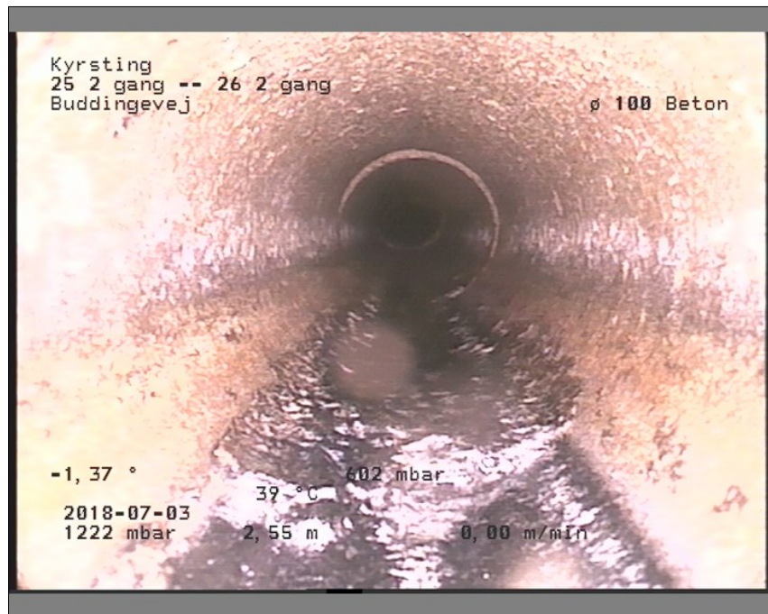
Foto: 25 2 gang-26 2 gang1006054-29-05-18_A.JPG, Medie #: De Engelske _0 1,77m, Aflejring klasse 1, fra urref 5 til urref 7, Hårde materialer, Start
