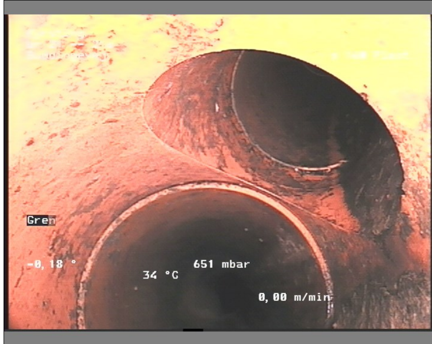
Foto: br 21-21a13510310-29-05-18_A.JPG, Medie #.: De Engelske _0, 00:01:01 13,49m, Grenrør klasse 0, urref 3
