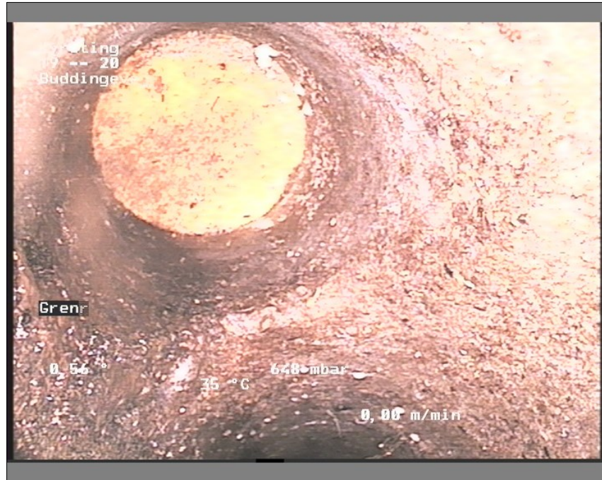
Foto: 19-2012564324-29-05-18_A.JPG, Medie #:: De Engelske _0, 00:05:29 56,45m, Grenrør klasse 0, urref 9, Stiktilslutning er afproppet
