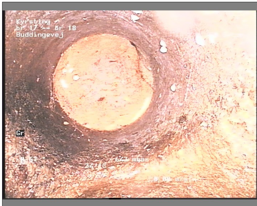
Foto: br 17-br 1811594025-29-05-18_A.JPG, Medie #: De Engelske _0, 00:07:53 20,87m, Grenrør klasse 0, urref 10, Stiktilslutning er afproppet / udgig til jord
