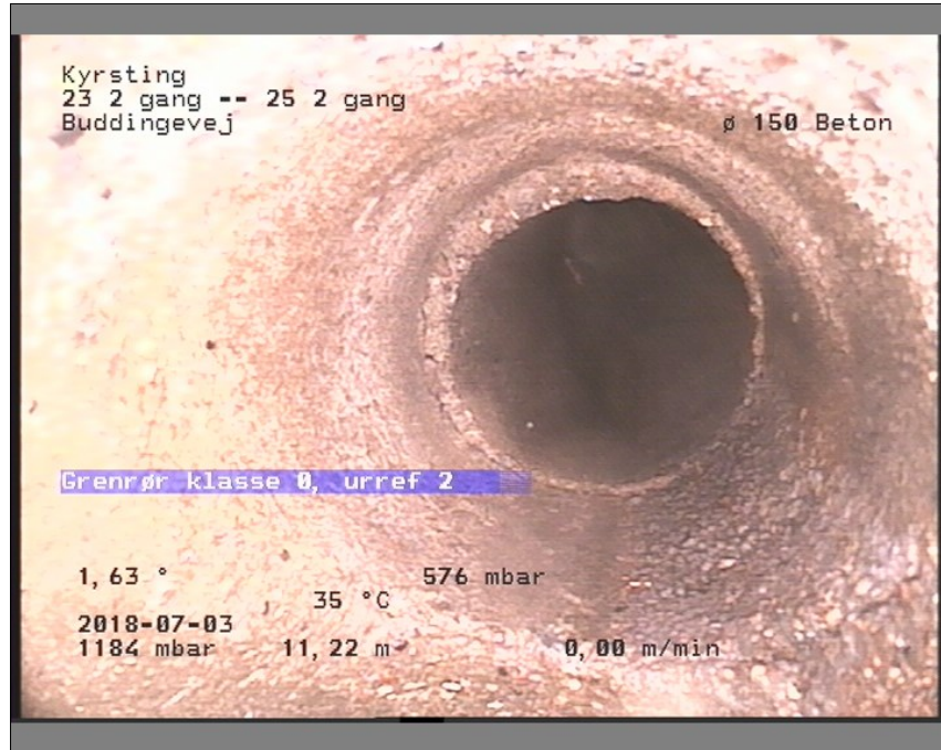
Foto: 23 2 gang-25 2 gang09260410-29-05-18_A.JPG, Medie #: De Engelske _0, 00:03:26 11,22m, Grenrør klasse 0, urref 2
