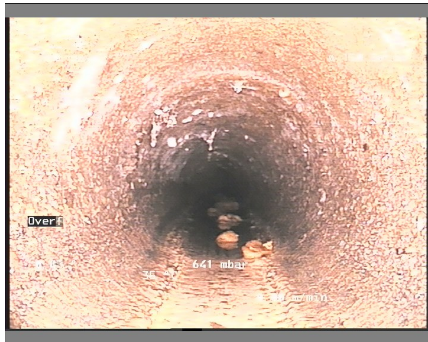
Foto: 16-1711271423-29-05-18_A.JPG, Medie #:: De Engelske _0, 00:00:37 16,66m, Overfladebeskadigelse klasse 3, fra urref 01 til urref 12, Stop
