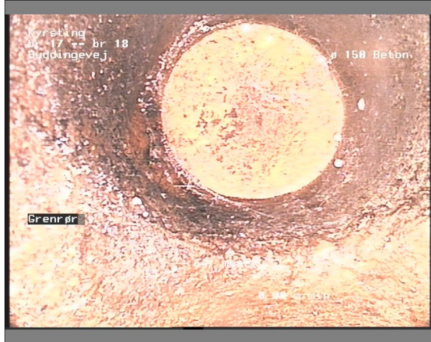
Foto: br 17-br 1811502117-29-05-18_A.JPG, Medie #: De Engelske _0, 00:05:14 13,94m, Grenrør klasse 0, urref 10, Stiktilslutning er afproppet
