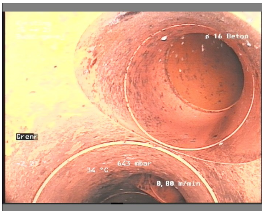
Foto: 15-2113365118-29-05-18_A.JPG, Medie #:: De Engelske _0, 00:05:25 24,83m, Grenrør klasse 0, urref 3
