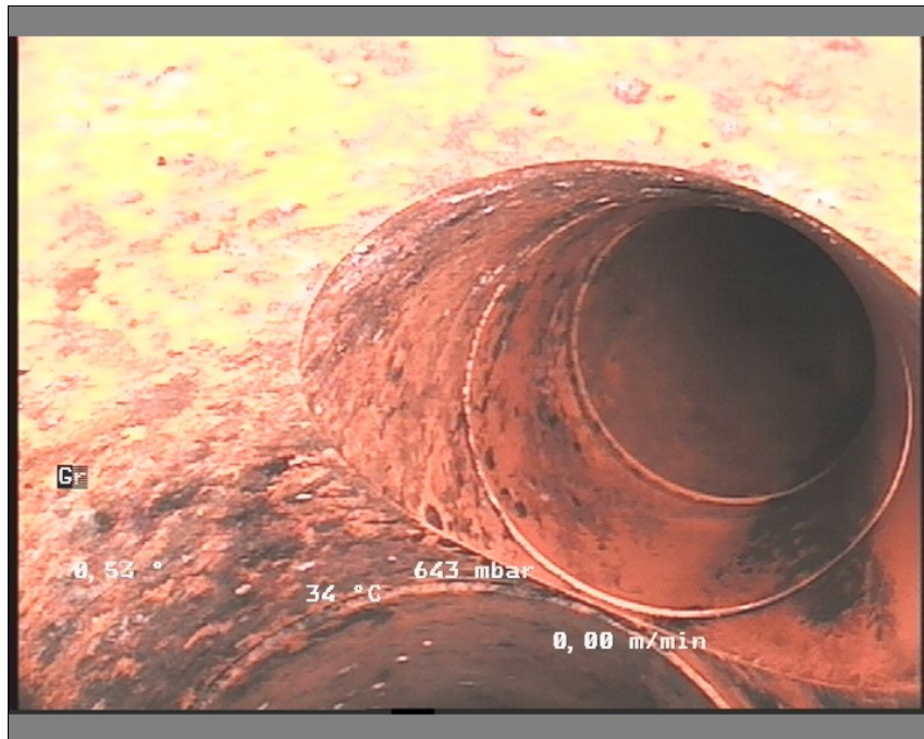
Foto: 15-2113370819-29-05-18_A.JPG, Medie #:: De Engelske _0, 00:05:35 25,01m, Grenrør klasse 0, urref 3
