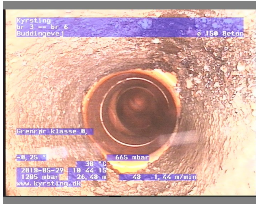
Foto: br 3-br 610442510-29-05-18_A.JPG, Medie #:: De Engelske _0, 00:07:36 26,45m, Grenrør klasse 0, urref 3
