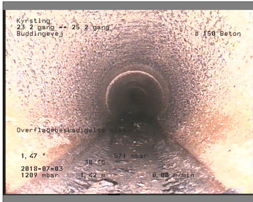
Foto: 23 2 gang-25 2 gang0859034-29-05-18_A.JPG, Medie #: De Engelske _0, 00:00:50 1,42m, Overfladebeskadigelse klasse 3, fra urref 1 til urref 3, Start
