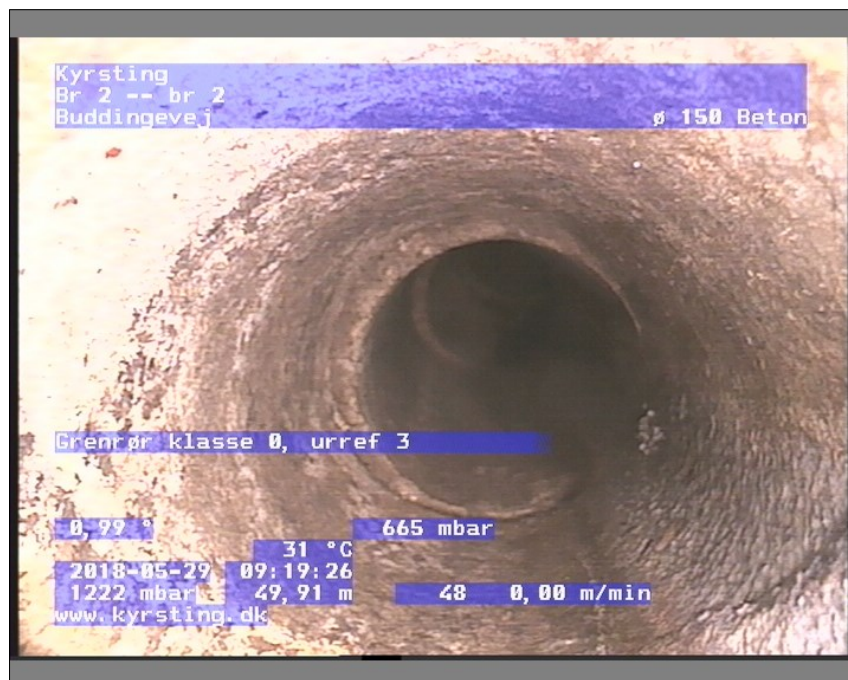
Foto: Br 2-br 209193629-29-05-18_A.JPG, Medie #:: De Engelske _0, 00:01:41 49,91m, Grenør klasse 0, urref 3
