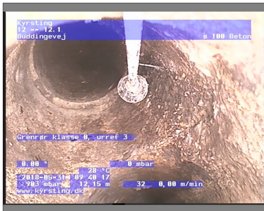
Foto: 12-12.109403312-29-05-18_A.JPG, Medie #.: De Engelske _0, 00:07:20 12,15m, Grenrør klasse 0, urref 3
