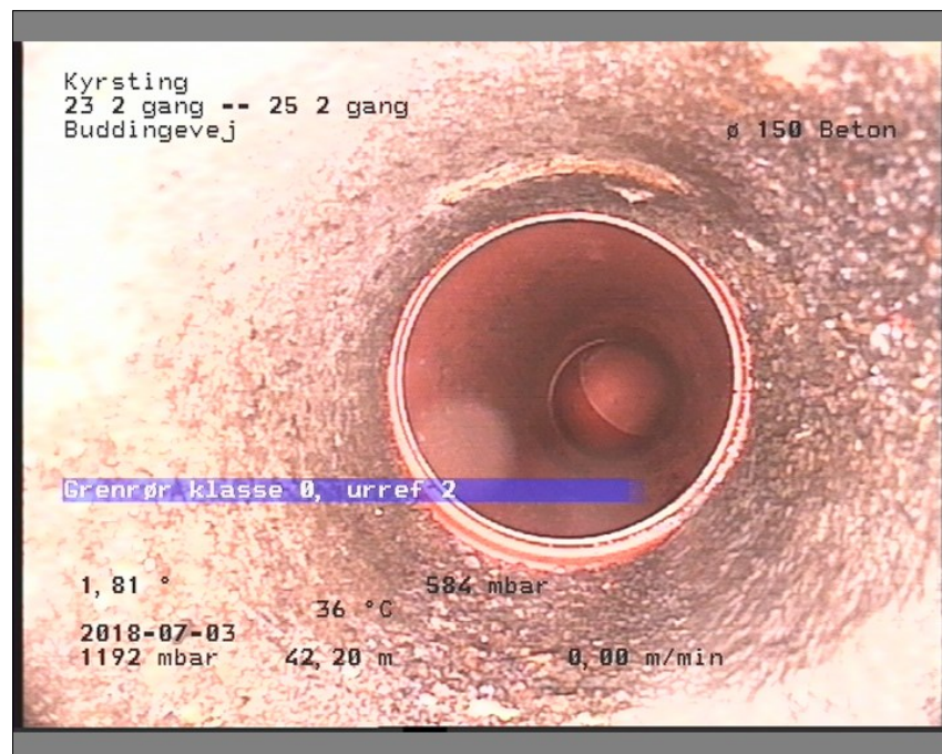
Foto: 23 2 gang-25 2 gang09380126-29-05-18_A.JPG, Medie #: De Engelske _, 00:11:29 42,2m, Grenrør klasse 0, urref 2
