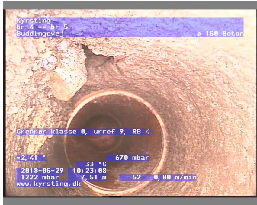
Foto: br 4-br 51023185-29-05-18_A.JPG, Medie #:: De Engelske _0, 00:02:47 7,51m, Grenrør klasse 0, urref 9 / RB 4 i gren
