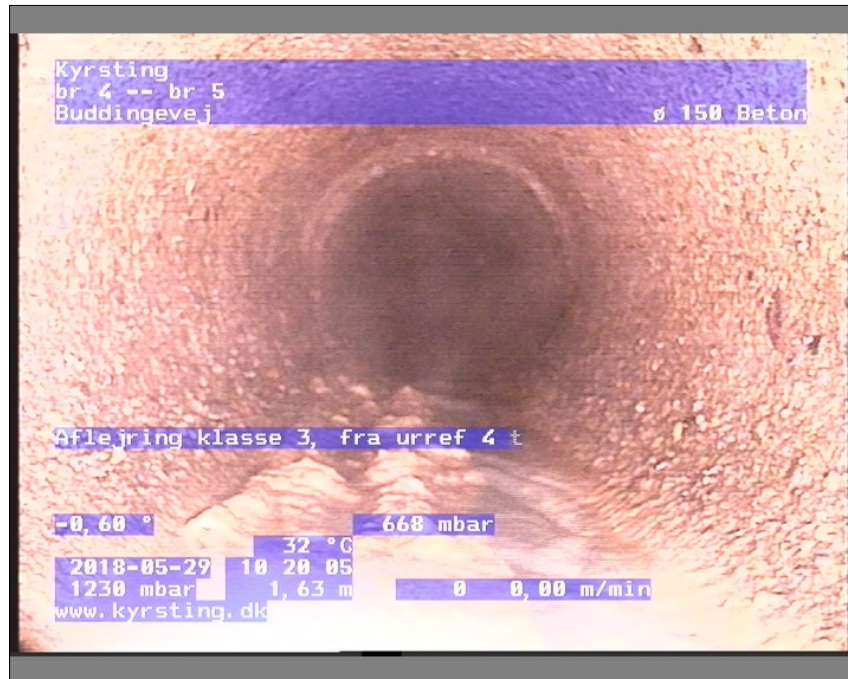
Foto: br 4-br 51020153-29-05-18_A.JPG, Medie #:: De Engelske _0, 00:00:35 1,63m, Aflejring klasse 3, fra urref 4 til urref 8, Hårde materialer, Start
