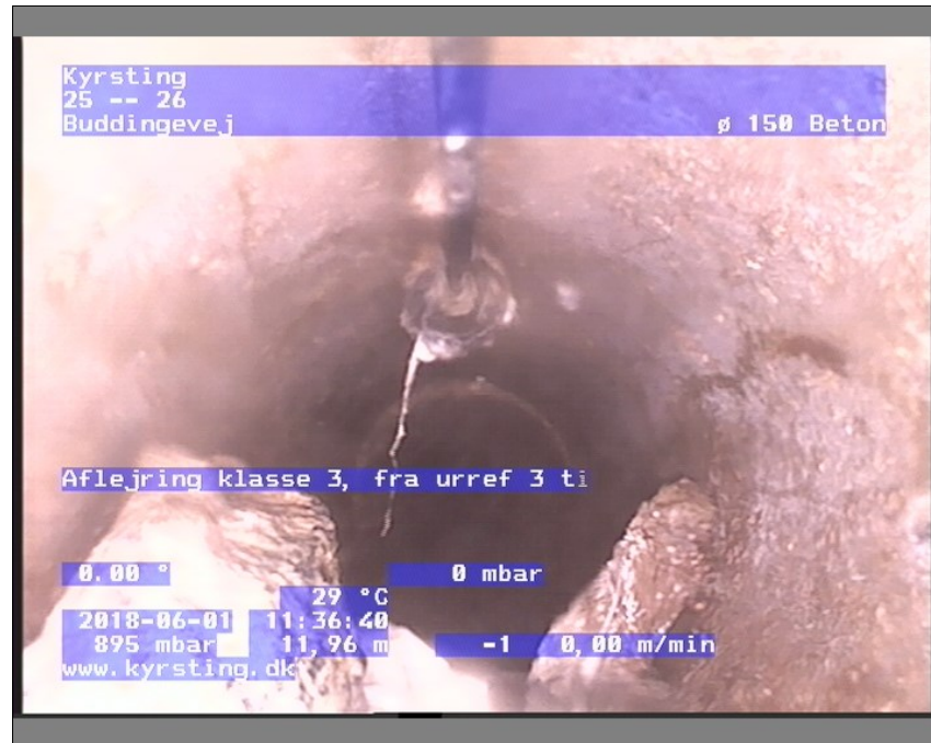
Foto: 25-2611365712-29-05-18_A.JPG, Medie #:: De Engelske _0, 00:05:49 11,96m, Aflejring klasse 3, fra urref 3 til urref 9, Sand/Grus
