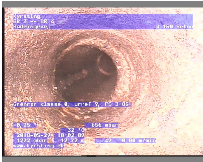
Foto: BR 3-BR 41002197-29-05-18_A.JPG, Medie #: De Engelske _0, 00:03:12 12,72m, Grenrør klasse 0, urref 9 / FS 3 OG RB 1 | GRENRØR
