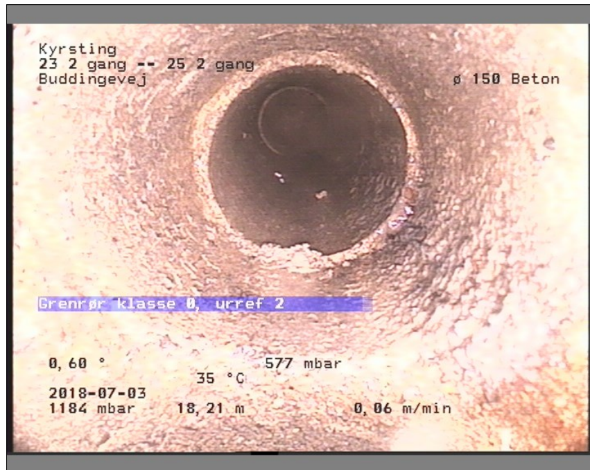
Foto: 23 2 gang-25 2 gang09275813-29-05-18_A.JPG, Medie #: De Engelske _0, 00:04:41 18,21m, Grenrør klasse 0, urref 2
