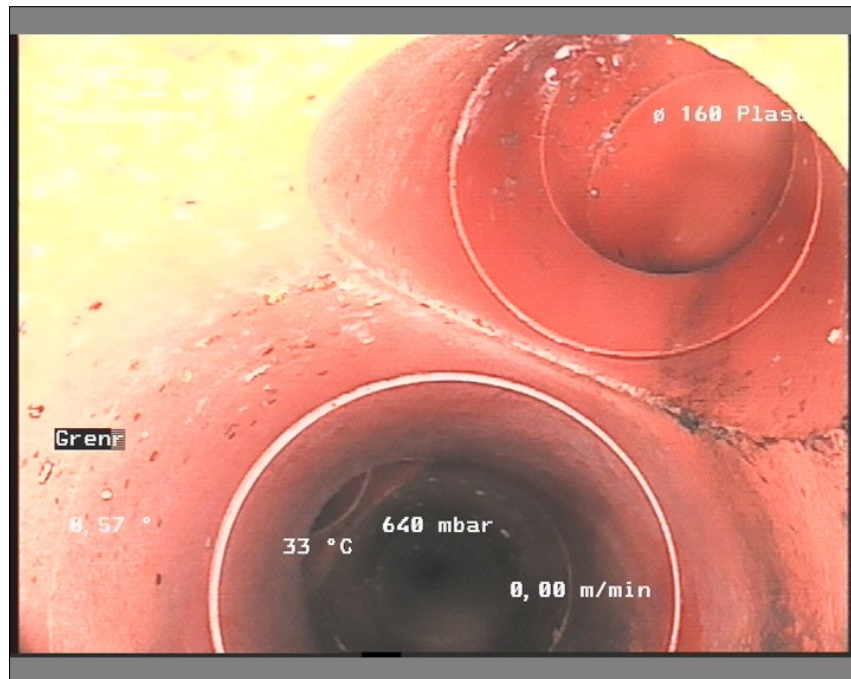
Foto: br 17-br 1811570720-29-05-18_A.JPG, Medie #: De Engelske _0, 00:06:31 16,37m, Grenrør klasse 0, urref 2
