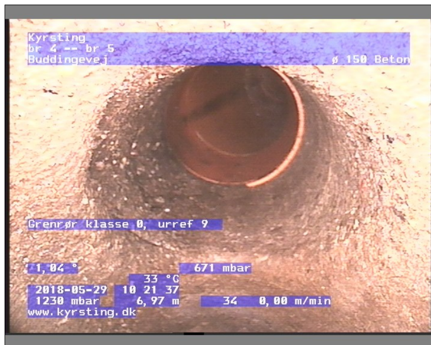
Foto: br 4-br 51021474-29-05-18_A.JPG, Medie #:: De Engelske _0, 00:01:53 6,97m, Grenrør klasse 0, urref 9
