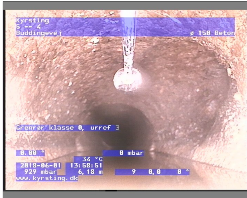
Foto: 4-51359074-29-05-18_A.JPG, Medie #:: De Engelske _0, 00:01:12 6,18m, Grenrør klasse 0, urref 3
