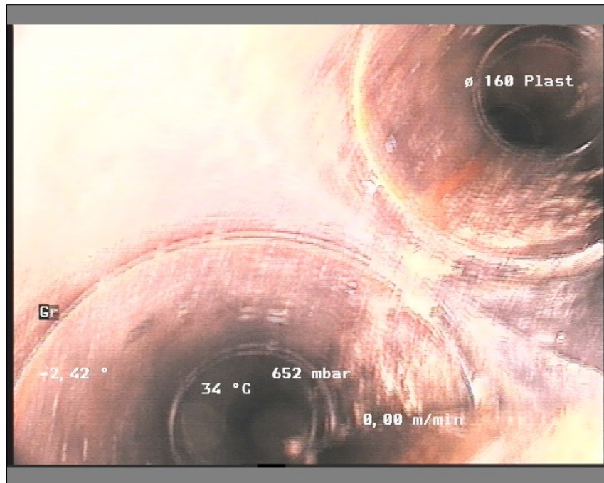
Foto: br 21-21a13570214-29-05-18_A.JPG, Medie #: De Engelske _0, 00:04:01 19,99m, Grenrør klasse 0, urref 3
