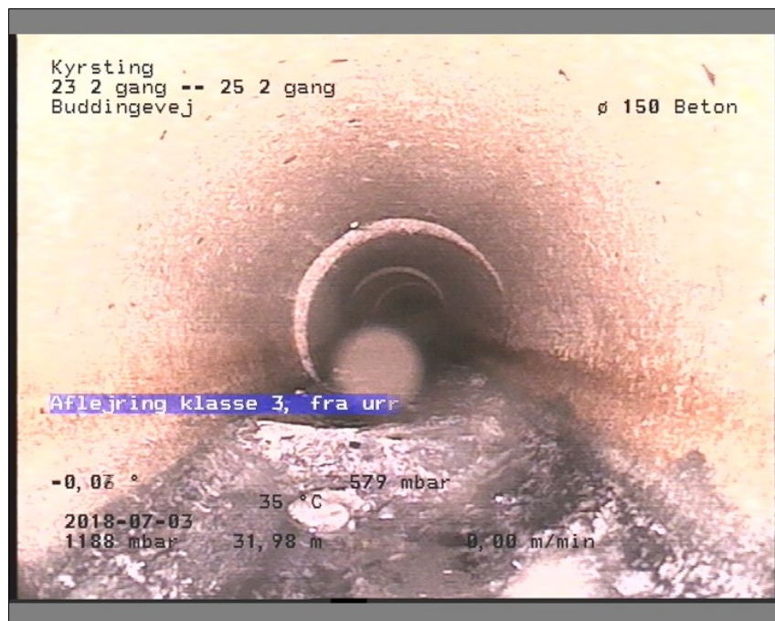
Foto: 23 2 gang-25 2 gang09332618-29-05-18_A.JPG, Medie #: De Engelske _0, 00:08:31 31,98m, Aflejrning klasse 3, fra urref 5 til urref 8, Hårde materialer, Start
