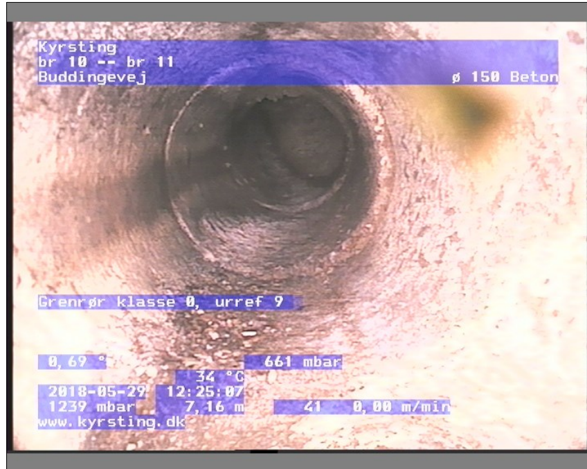
Foto: br 10-br 111225174-29-05-18_A.JPG, Medie #.: De Engelske _0, 00:02:15 7,16m, Grenrør klasse 0, urref 9
