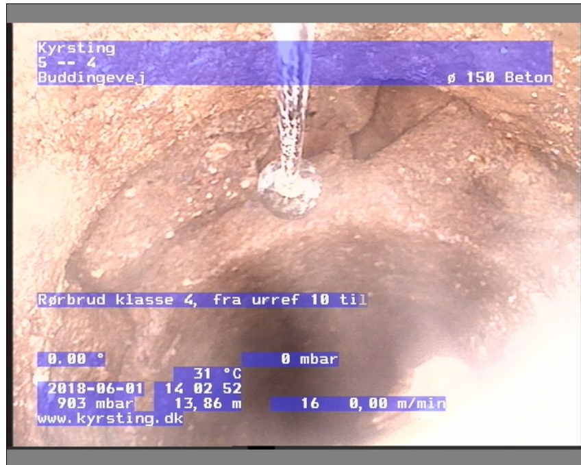
Foto: 4-514030814-29-05-18_A.JPG, Medie #.: De Engelske _0, 00:03:36 13,86m, Rørbrud klasse 4, fra urref 10 til urref 4, Brud
