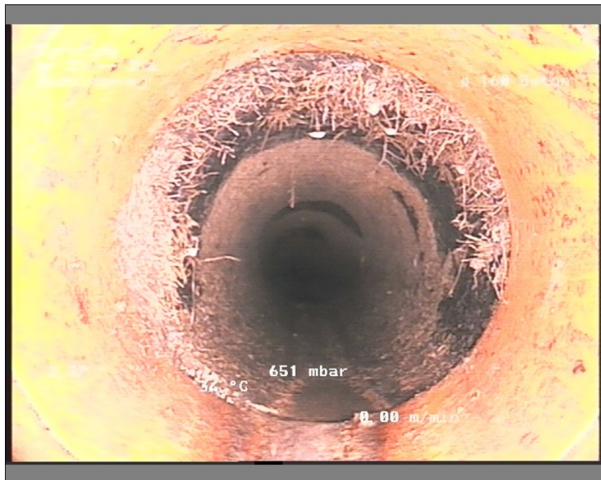
Foto: br 21-21a13543211-29-05-18_A.JPG, Medie #.: De Engelske _0, 00:02:13 14,36m, Konstruktionsændring klasse 3, Dimensionsændring, Materialeændring
