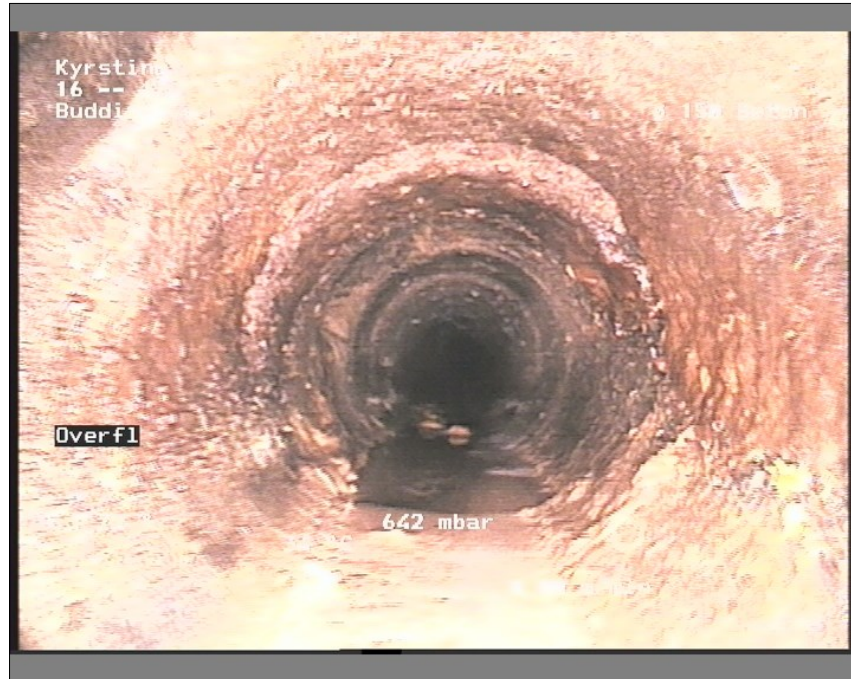
Foto: 16-1711295530-29-05-18_A.JPG, Medie #:: De Engelske _0, 00:00:37 22m, Overfladebeskadigelse klasse 3, fra urref 1 til urref 12, Start
