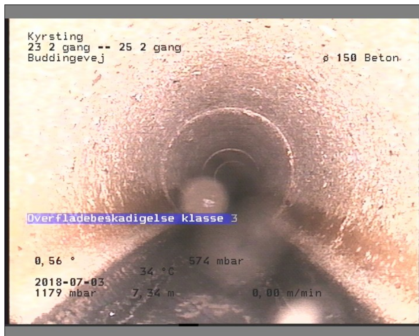
Foto: 23 2 gang-25 2 gang0924288-29-05-18_A.JPG, Medie #: De Engelske _0, 00:02:22 7,34m, Overfladebeskadigelse klasse 3, fra urref 01 til urref 03, Stop
