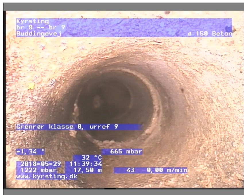
Foto: br 8-br 911394414-29-05-18_A.JPG, Medie #:: De Engelske _0, 00:04:36 17,5m, Grenrør klasse 0, urref 9
