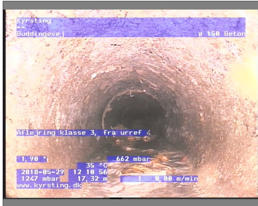
Foto: br 9-br1012110716-29-05-18_A.JPG, Medie #:: De Engelske _0, 00:06:14 17,32m, Aflejring klasse 3, fra urref 4 til urref 7, Hårde materialer, Fastsiddende, Start
