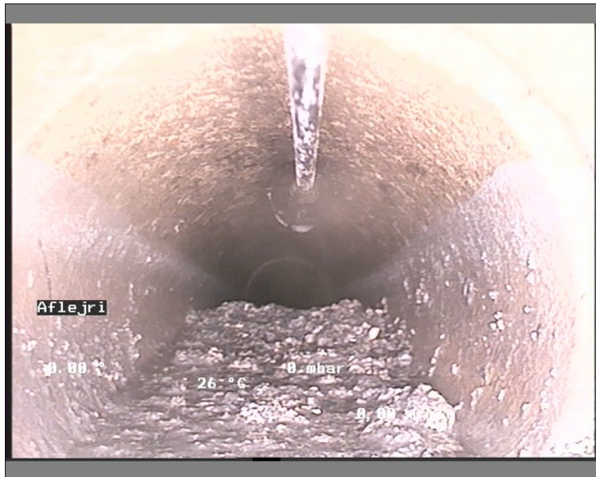
Foto: 14-130927424-29-05-18_A.JPG, Medie #.: De Engelske _0 2,08m, Aflejring klasse 3, fra urref 2 til urref 9, Sand/Grus, Aflejring af anden type
