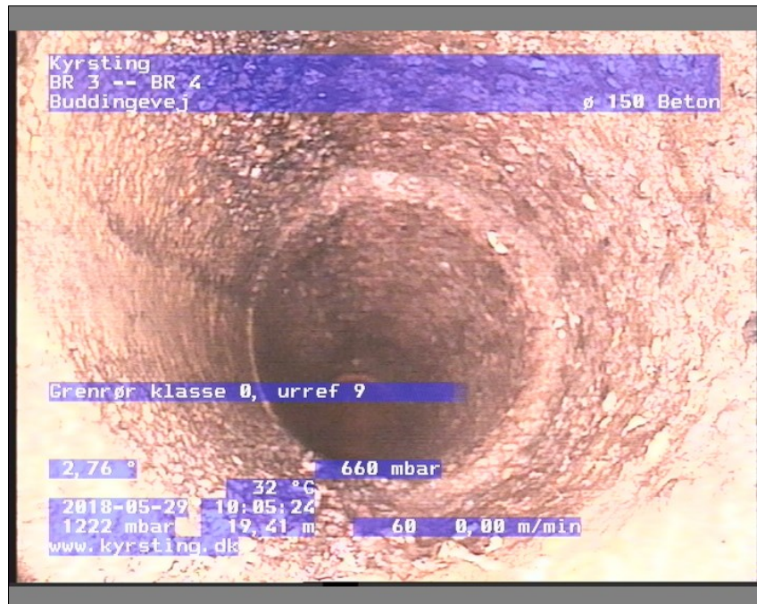
Foto: BR 3-BR 410053413-29-05-18_A.JPG, Medie #:: De Engelske _0, 00:05:27 19,41m, Grenrør klasse 0, urref 9
