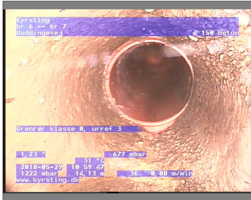
Foto: br 6-br 71059579-29-05-18_A.JPG, Medie #:: De Engelske _0, 00:06:02 14,13m, Grenrør klasse 0, urref 3
