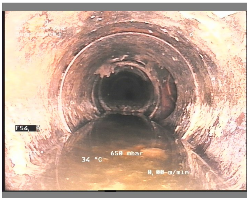
Foto: br 21-21a14001323-29-05-18_A.JPG, Medie #.: De Engelske _0, 00:05:51 26,91m, FS4, Åben samling
