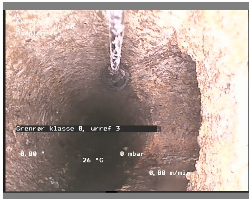
Foto: br 10-br 111334168-29-05-18_A.JPG, Medie #.: De Engelske _0, 00:02:58 19,22m, Grenrør klasse 0, urref 3
