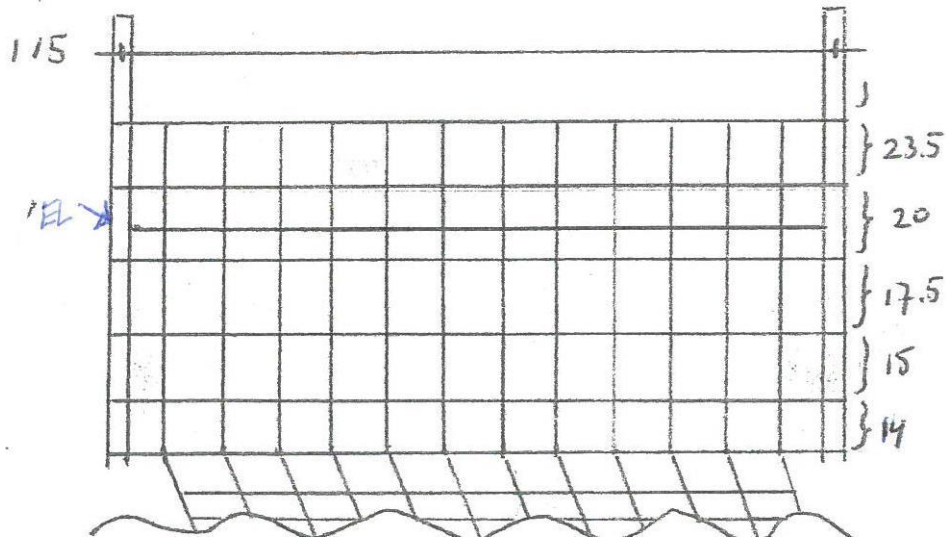
Billed 2 1 eltråd udvendigt 60-90 cm over jord og 1 eltråd øverst 115 cm over jord Derudover anbefales det at sætte en tråd indvendigt ca. 30 cm over jorden for at beskytte nethegn
