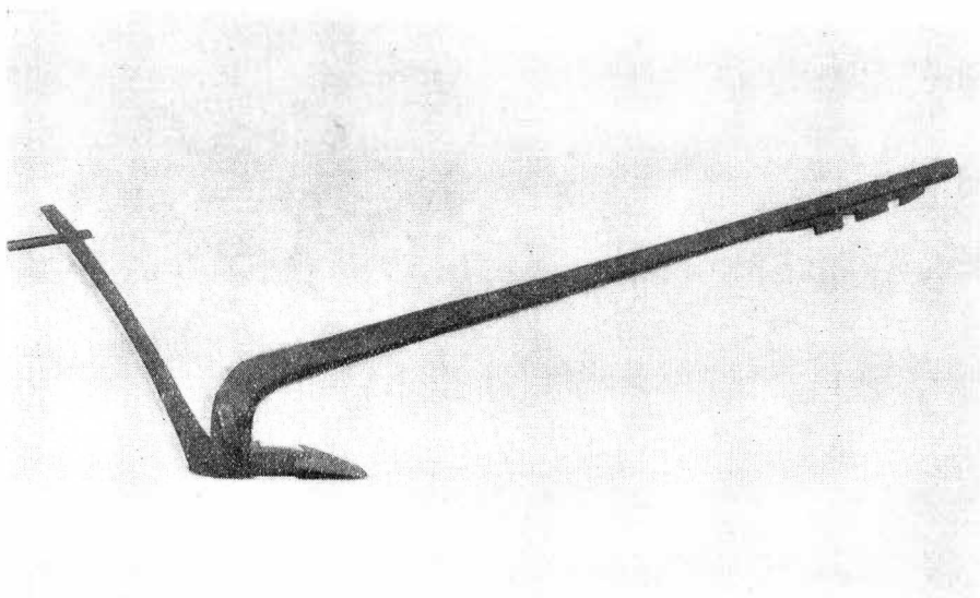
Fig. 4. Krok från Axvall, Norra Ving sn, Valle hd. L. 3,74 m. LM 24. Efter Jirlow 1951, fig. 95.
