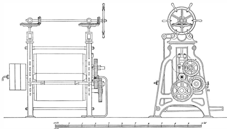
Glansmangel år 1888
