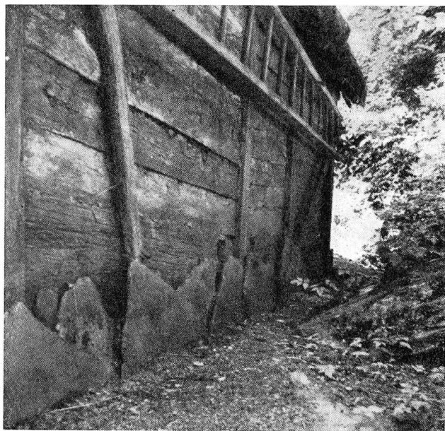
Parti av uthuslängans östvägg. Märk de tunna stenhällarna, avsedda att hindra vattenstänk mot väggens nedersta plankor. Foto Albert Sandklef.
