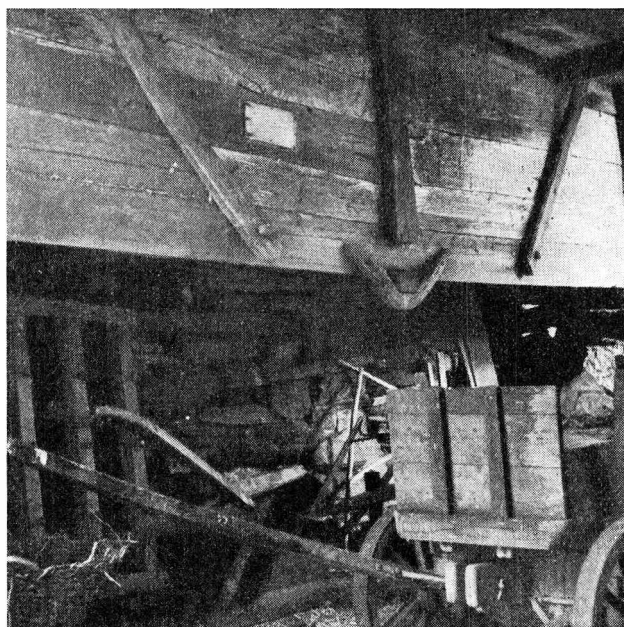
Från portskjulet. Märk den i texten beskrivna upphängningsanordningen för foderlogens golvbjälke och den på bilden synliga upphängningsanordningen för väggens syll. Foto. I. Vallin.
