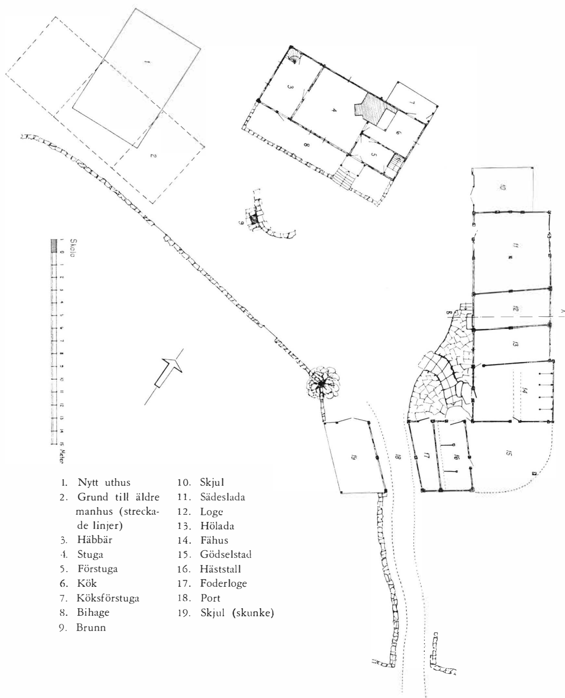
Planritning över Märkedal i Grimmaröd. Uppmätning och ritning av Albert Sandklef år 1952.
