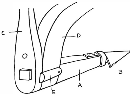
Fig. 2. Krok. Detalj av 1700-talsmodell från Västergötland. L. 0,56 m. A vise, B bill med tånge och ring, C bakståndare, D ås, E öra. U 81. Efter Jirllow 1948.
