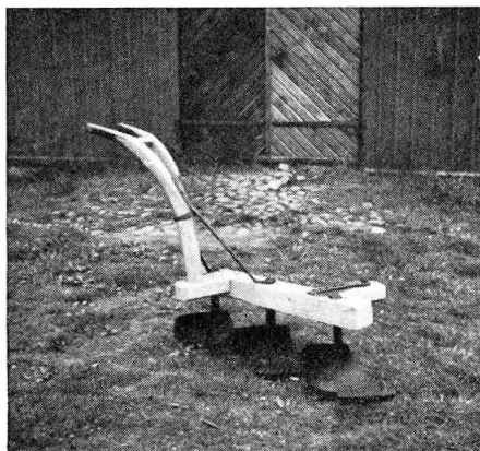
Fig. 29. Treskärig skumplog. Timmele sn, Redvägs hd. Fristads museum.
