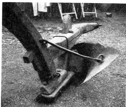
Fig. 22. Plog. Askims hd. L. 2,54. Bakståndaren upptill spräckt, nedtill med dubbelriktat knä, fäst med tränaror. Uddevalla museum.
