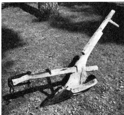
Fig. 13. Årder. L. 1,3 m. Ljushult sn, Kinds hd. Borås museum 7838.
