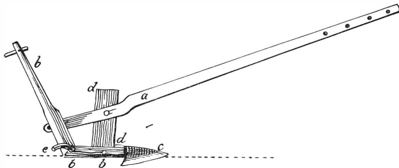
Fig. 8. Lågårder, krok: a krokåsa , bbb krokshuvud , c bil , dd värj . e öra. Vadsbo bd. Efter Berch-Bergman 1759.
