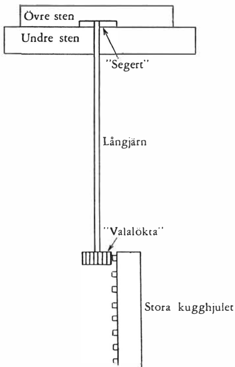
Ovanstående skiss visar hur kvarnen drevs.
