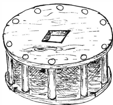
Valalökta. Kugghjul av trä med plåthylsor på pinnarna.
