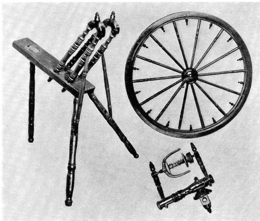
Spinnrocken består av tre huvuddelar: stolen, hjulet och vingtyget.
