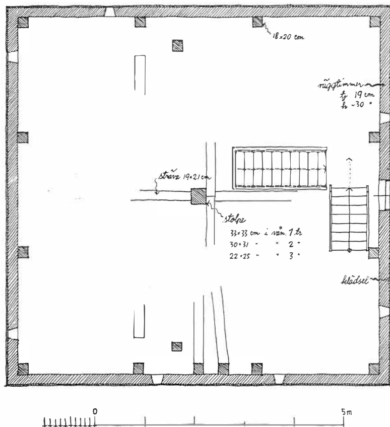
Uppmätning av Håksviks kyrktorn. Plan av vån. 2 tr. upp. Arkitekt Svante Paulson 1938.
