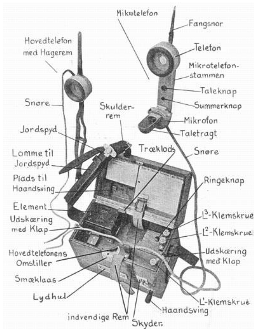
Felttelefon E.
