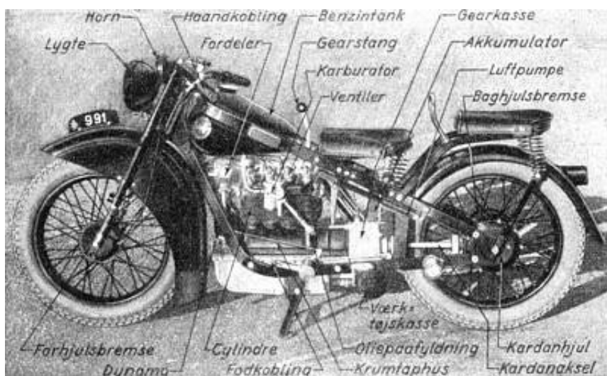
Nimbus motorcykel.
