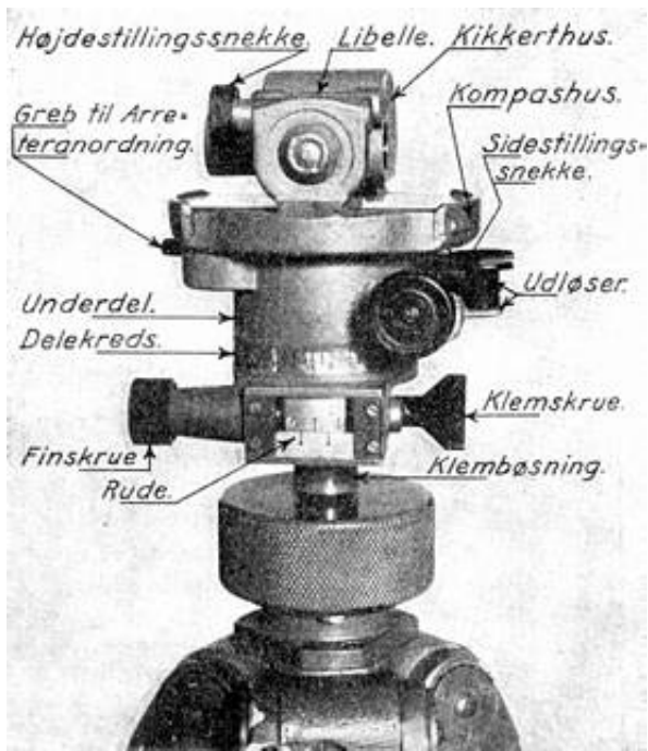
Vinkelmåler M.1924
