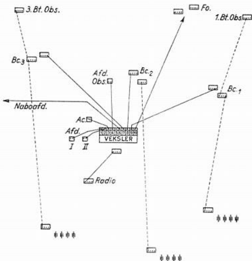
Principskitse, afdelingens telefonnet
