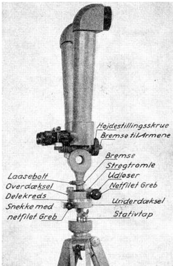
Reliefkikkert M.1924
