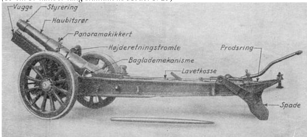
15 cm L/17 S.H. M.1923 (15 cm 17 kaliber lang stålhaubits Model 1923)
