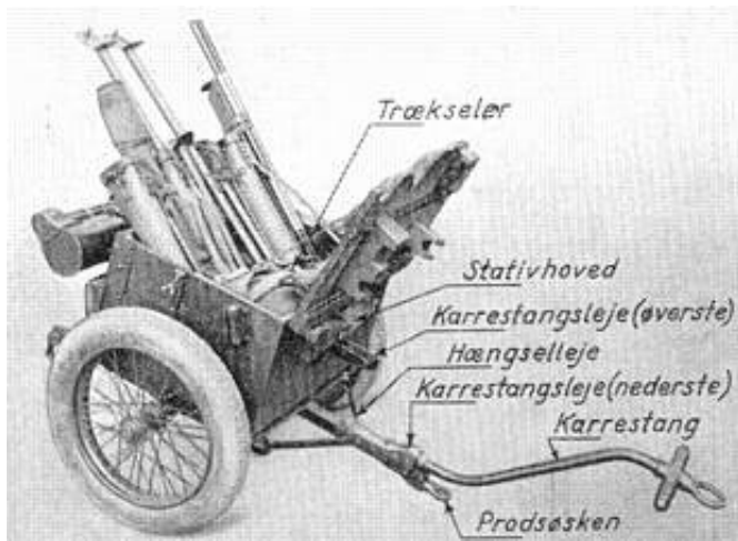
Maskingeværkarre M.1932. Fra Kilde 2.
