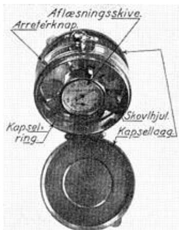
Vindmåler M.1930.
