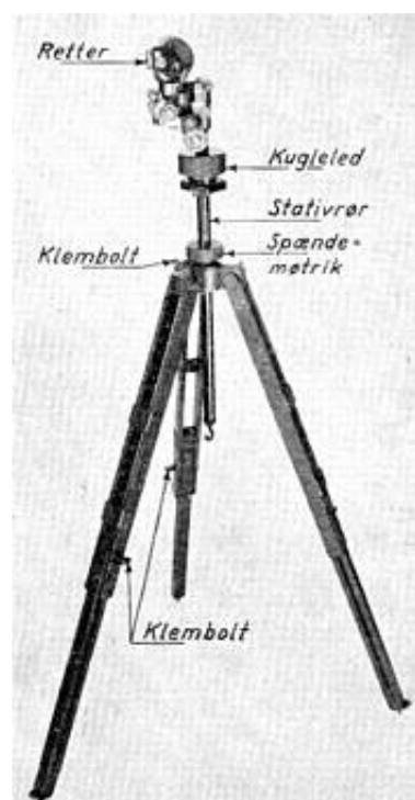
Retter M.1930. Fra Kilde 2.
