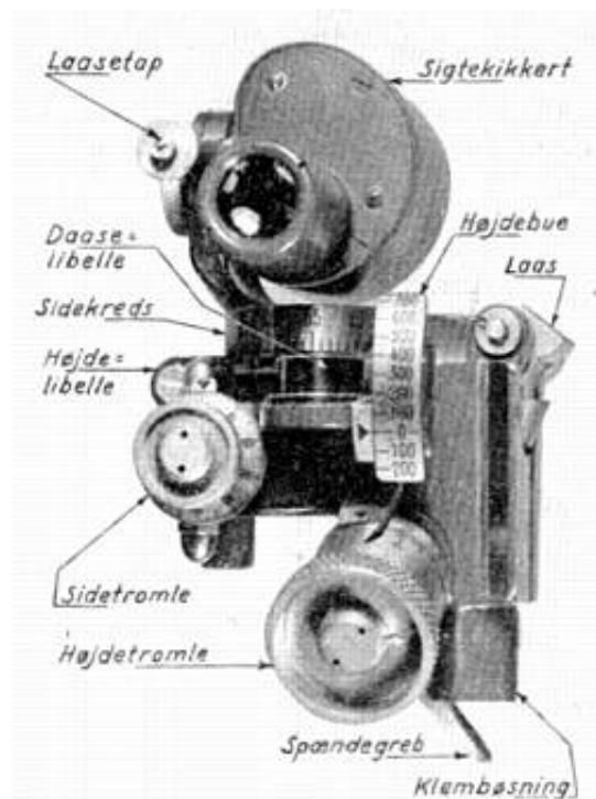
Retter M.1930. Fra Kilde 2.
