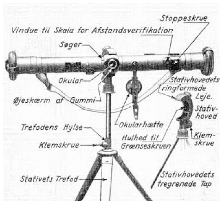
Afstandsmåler M.1915.
