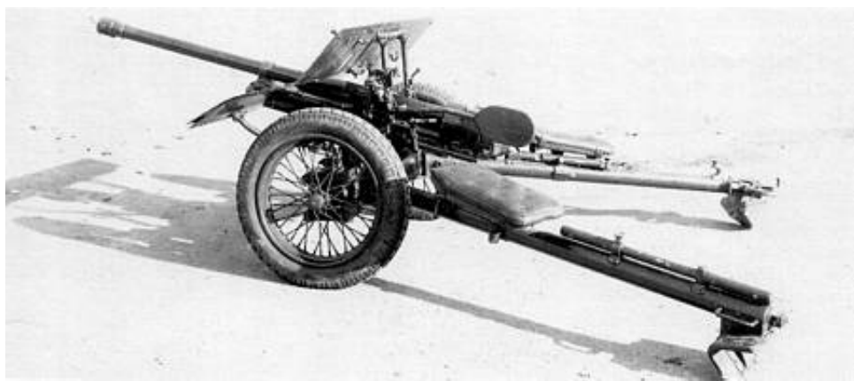
37 mm fodfolkskanon M.1937 2 ).
