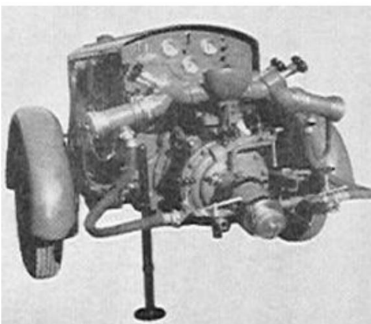
Pulvérisateur traîné suédois (type API 120). De la caserne de pompiers de Gysinge.
