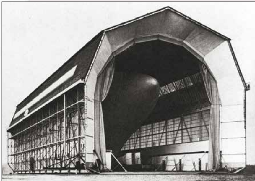
Den første drejelige luftskibshal blev bygget i Berlin-Biersdorf i 1911. Drejeanordningen er ikke synlig på billedet. Foto fra Wikipedia.
