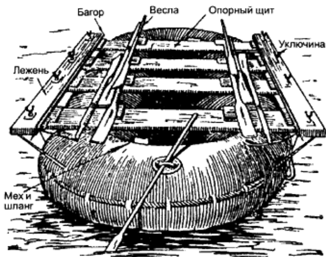
Gummibåd af typen A-3
