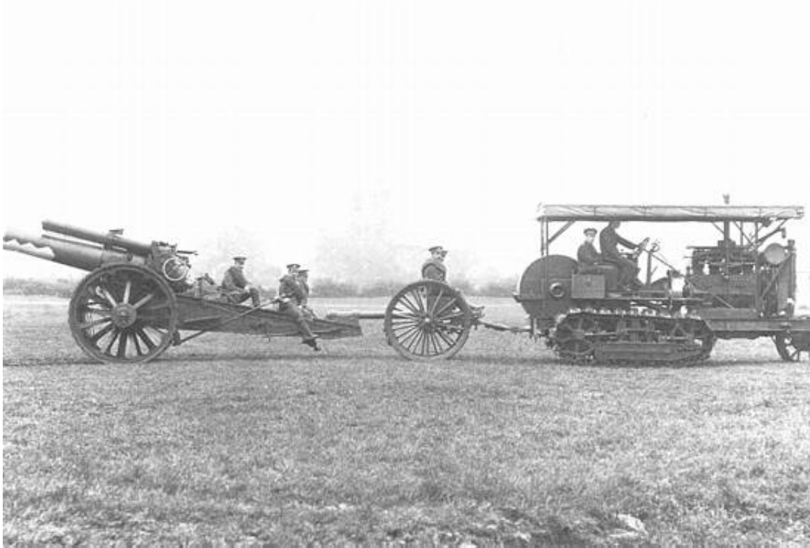
Holt 75-h.p. Petrol Tractor trækker en 8" haubits, Mk 1-5. Fra Kilde 3.
