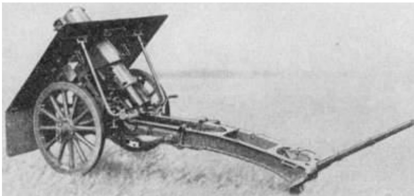
7,5 cm bjergkanon (Skoda) Model 1928.
