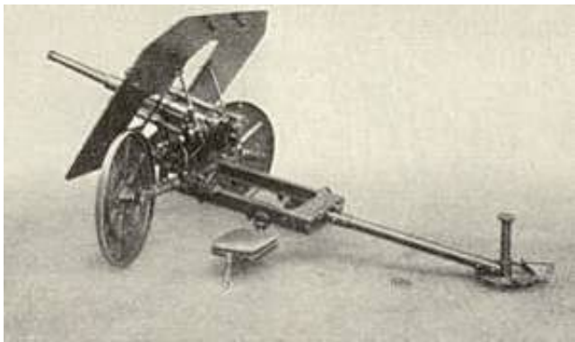
3,7 cm panserværnskanon (Skoda). Ved i stedet at montere et udskifteligt kanonrør - kaliber 7 cm - kunne pjecen fungere som en infanterikanon. Skudvidden var da 2,5 km.
