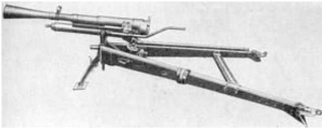
3,7 cm infanterikanon (fransk) Model 1916. Skudvidde: 2,5 km.
