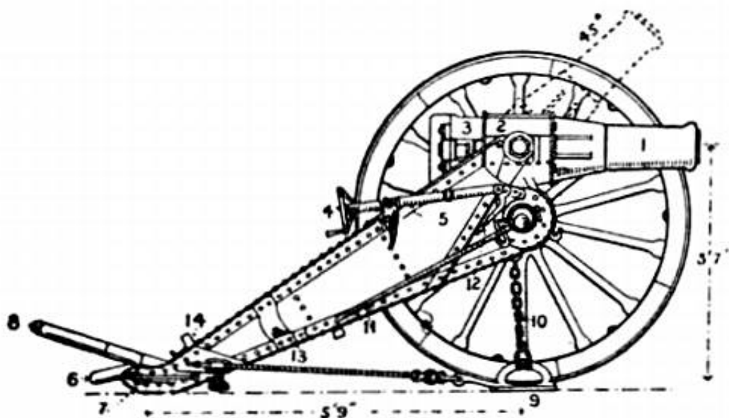
BL 5-inch Field Howitzer. Fra Kilde 8.
