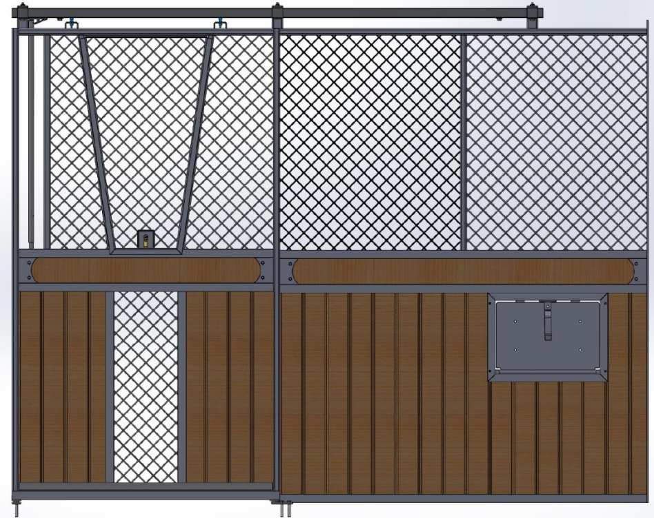
Ruter Knekt - Galvad med granplank och dekorationsbräda samt öppningsbar lucka i fronten som kan hakas av, ljusinsläpp i front samt vippkrubba.
