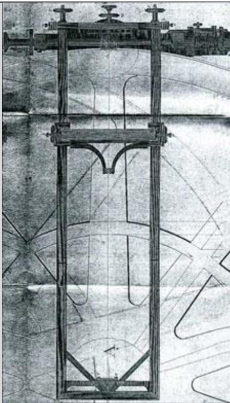
Slæden på Ramsdens inddelingsmaskine.
