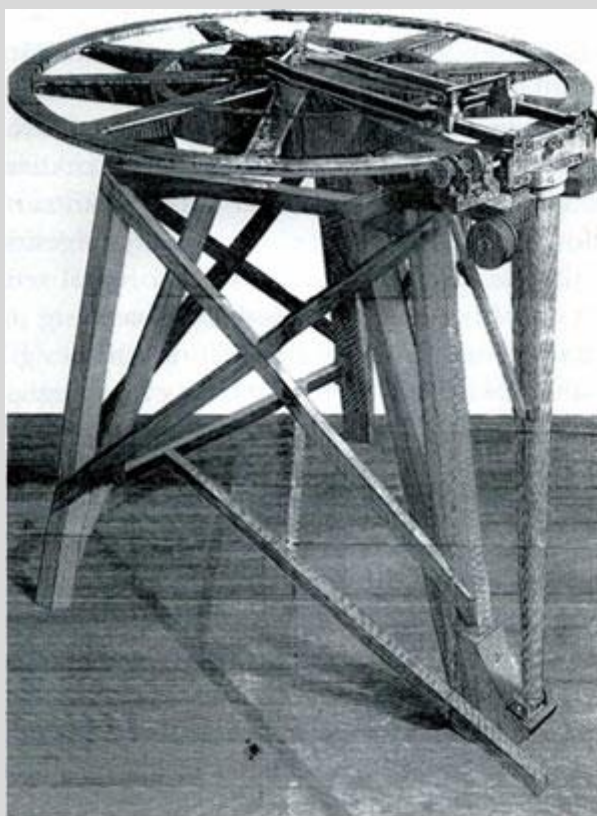
Ill.7. Ramsdens inddelingsmaskine.
