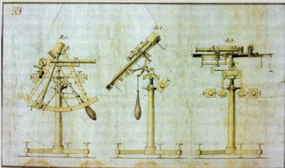
Ill.5-6. Jesper Bidstrups sekstant.
