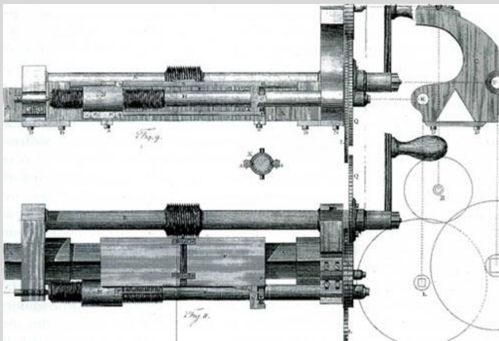
Ill.8. Ramsdens drejebænk til skæring af gevind i den endeløse skrue.
