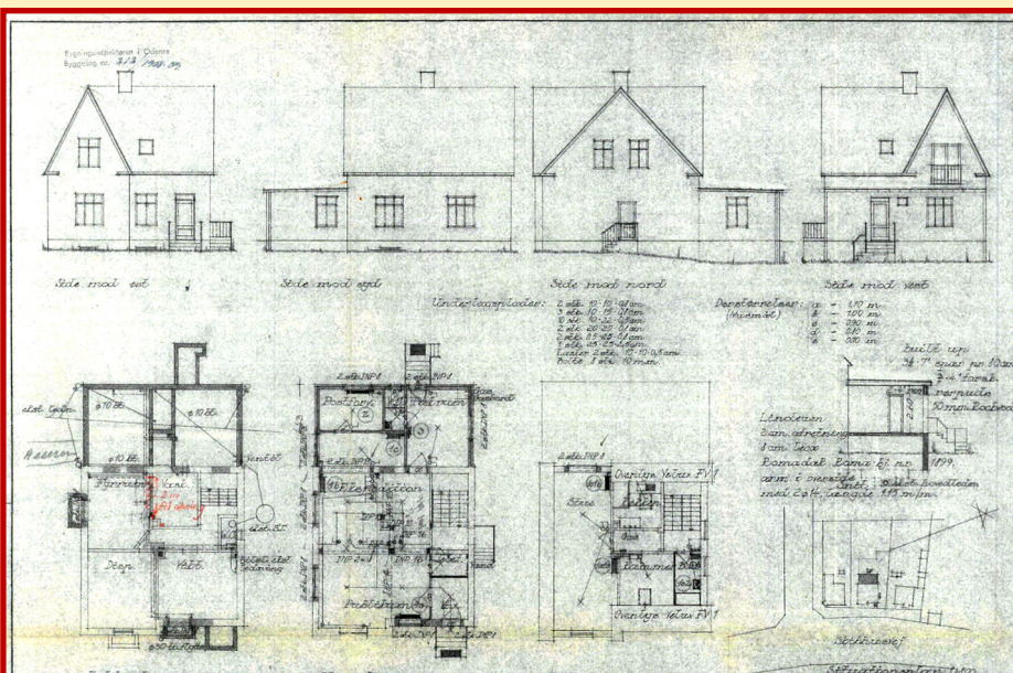
Tegninger af postbygningen på Skibhusvej 158 og herunder plan- og facadetegning af den nye postbygning fra 1979.
