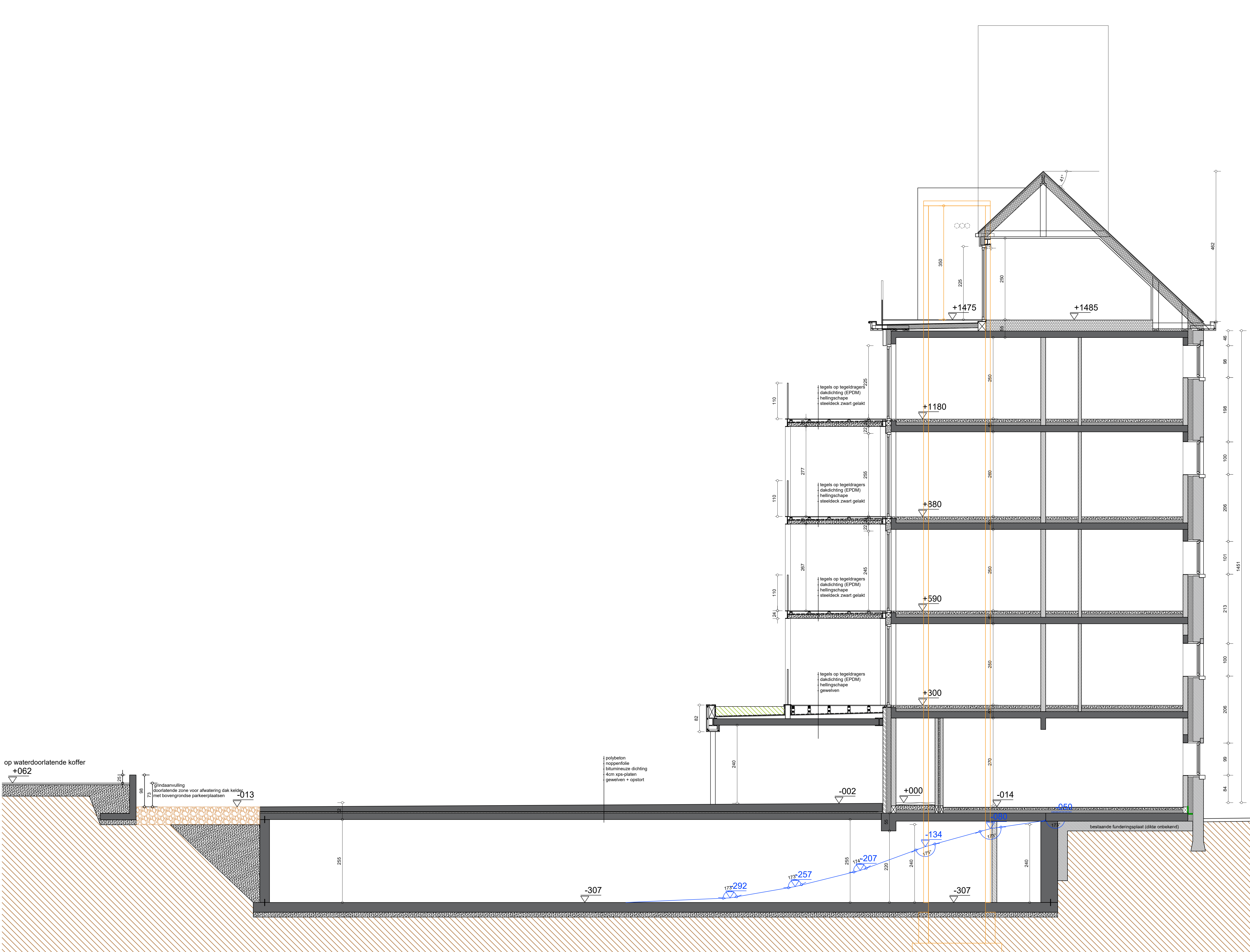
snede AA
