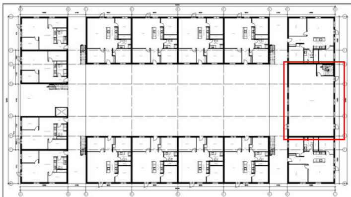
STUEPLAN
