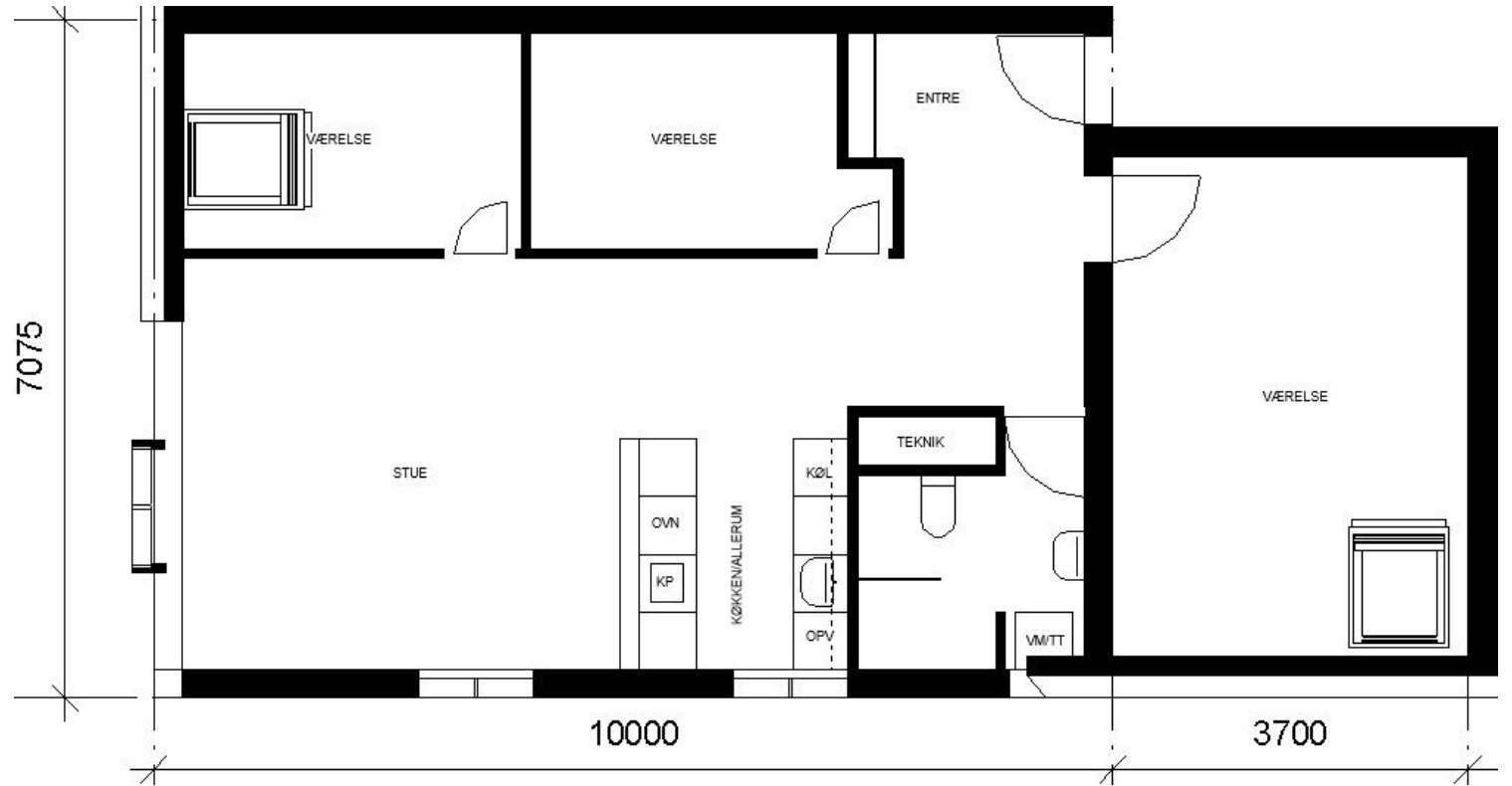
STUEPLAN
