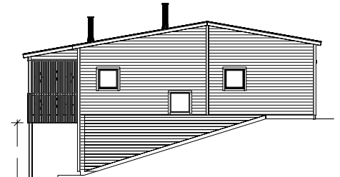
Fasad mot sydost
