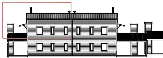
Fasad mot nordost
