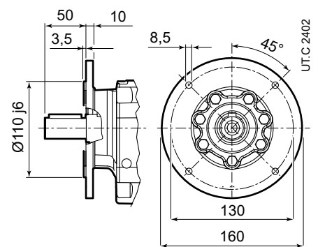
F216 Ø 160
