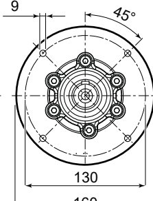
F316 Ø 160
