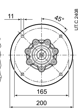
F420 Ø 200
