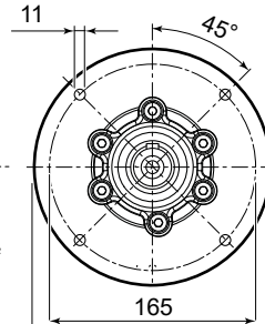
F320 Ø 200
