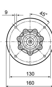
F416 Ø 160
