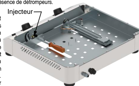
Brûleur Fusion 75 avec bague d'air
